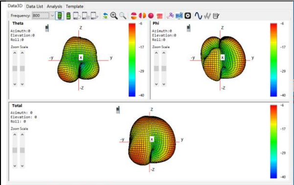
Main: 800Mhz
