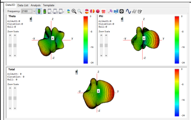
Aux: 2160Mhz
