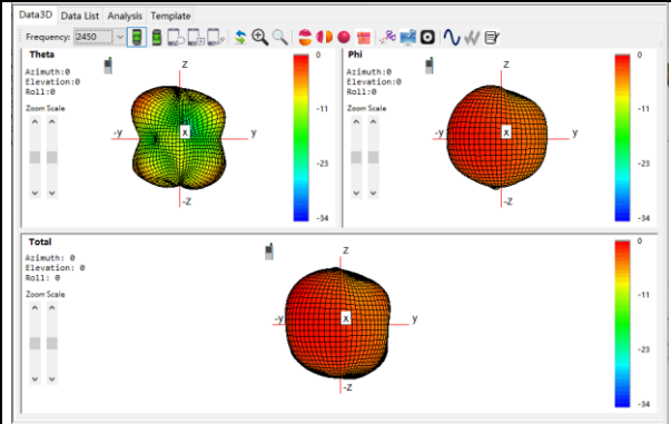
G/W/B: 2450Mhz
