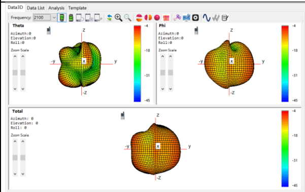
Main: 2100Mhz
