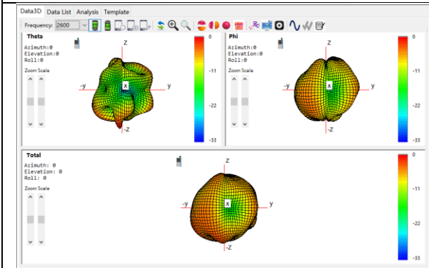
Aux: 2600Mhz
