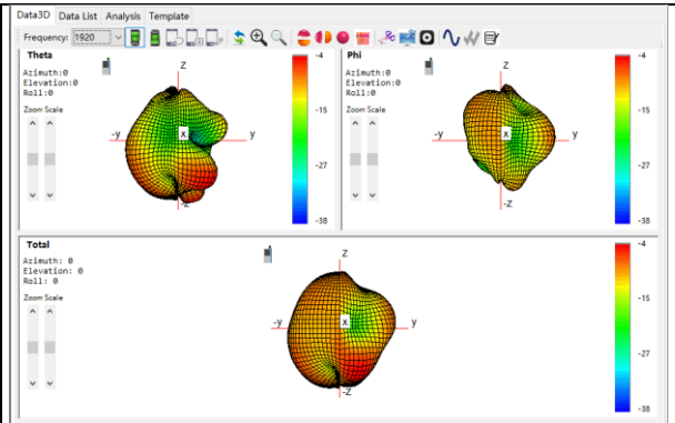
Aux: 1920Mhz
