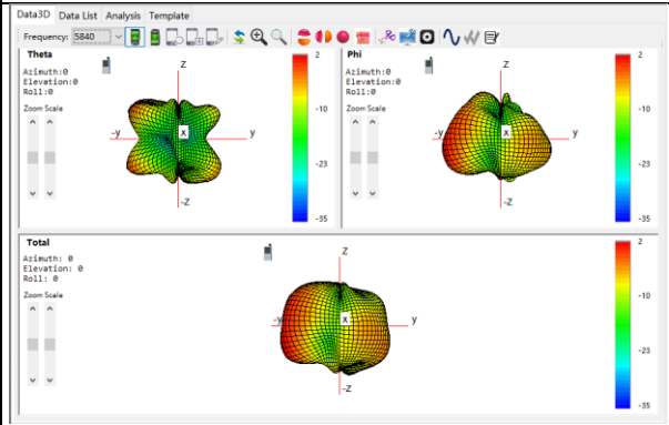
G/W/B: 5840Mhz
