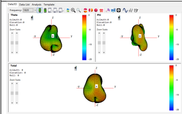
Aux: 1820Mhz
