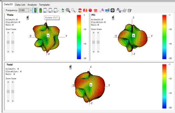
G/W/B: 5180Mhz
