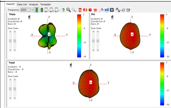
Main: 2600Mhz
