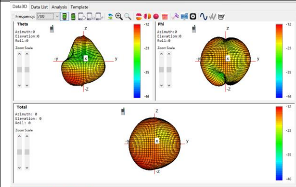
Main: 700Mhz
