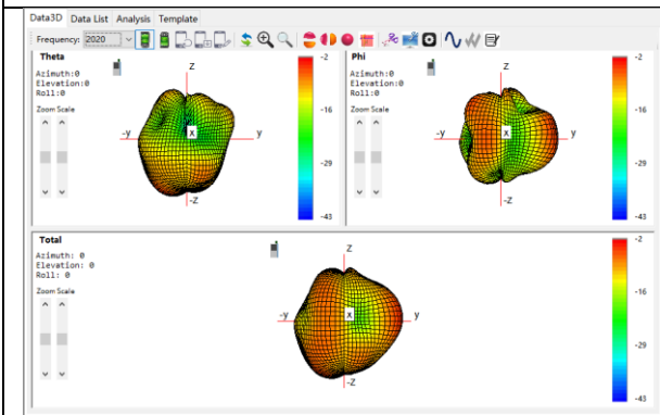
Aux: 2020Mhz
