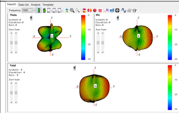
Main: 1900Mhz
