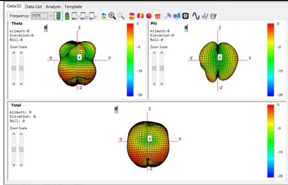
G/W/B: 1575Mhz
