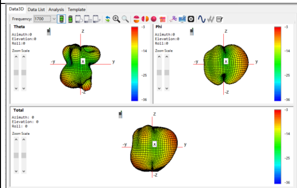
Main: 1700Mhz
