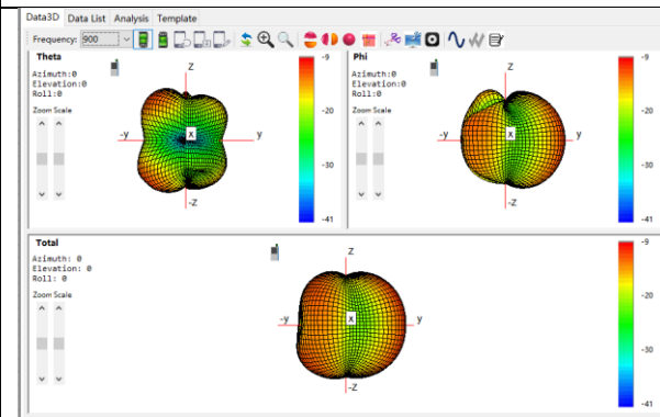
Main: 900Mhz
