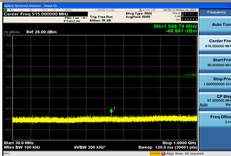
Band4-5MHz-QPSK-20375-1RB#0-30~1000MHz
