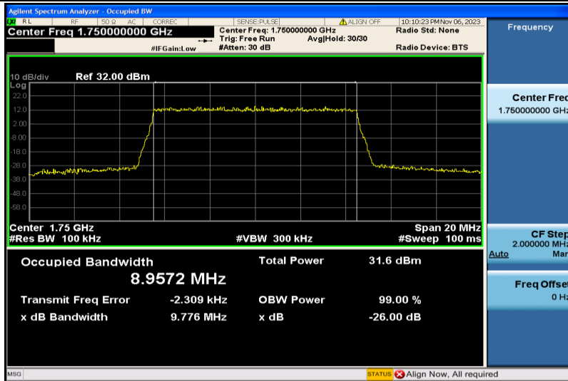
Band4-10MHz-QPSK-20350-50RB#0-8.9572
