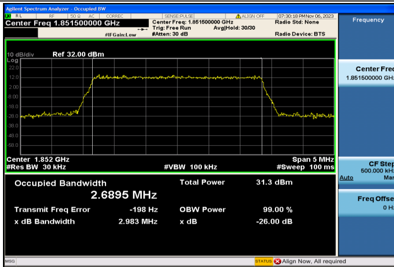
Band2-3MHz-QPSK-18615-15RB#0-2.6895
