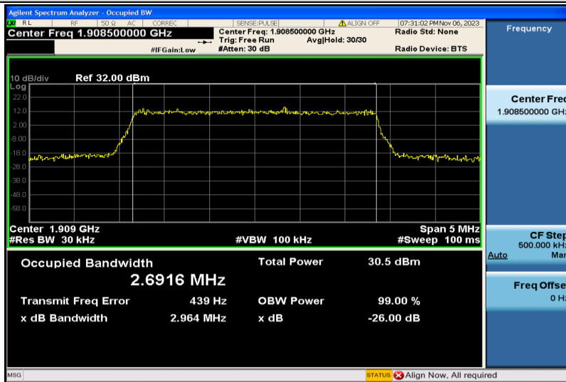
Band2-3MHz-QPSK-19185-15RB#0-2.6916
