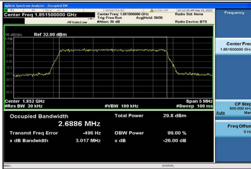
Band2-3MHz-QPSK-18615-15RB#0-2.6886
