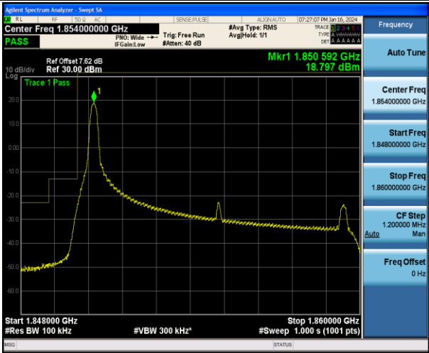
Band2_10MHz_QPSK_18650_1RB#0
