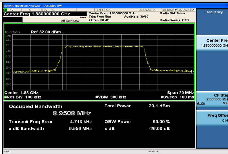
Band2-10MHz-16QAM-18900-50RB#0-8.9508
