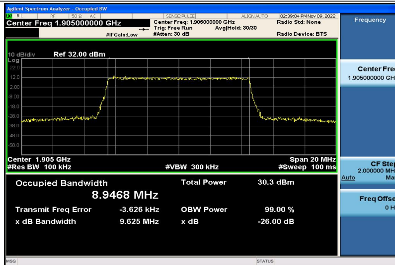
Band2-10MHz-QPSK-19150-50RB#0-8.9468
