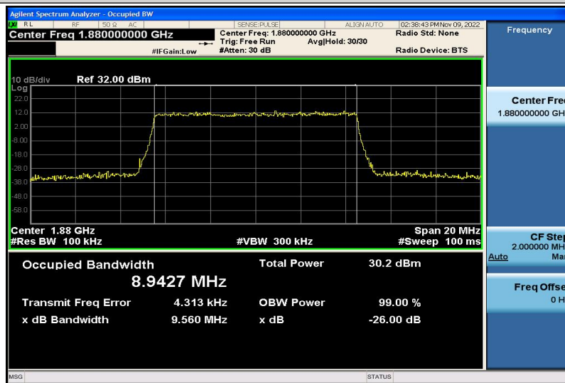
Band2-10MHz-QPSK-18900-50RB#0-8.9427
