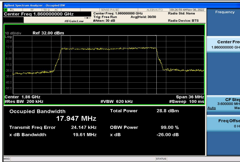
Band2-20MHz-QPSK-18700-100RB#0-17.947
