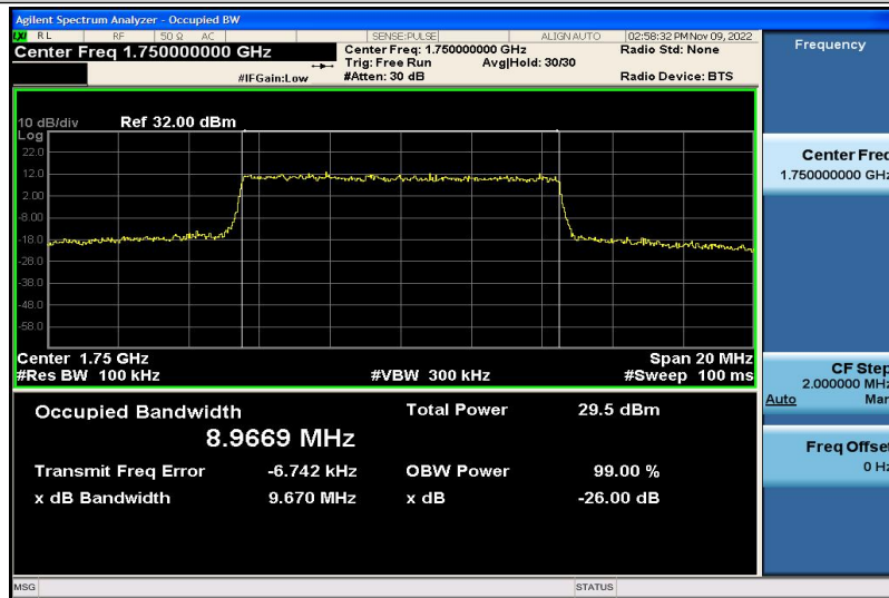
Band4-10MHz-QPSK-20350-50RB#0-8.9669
