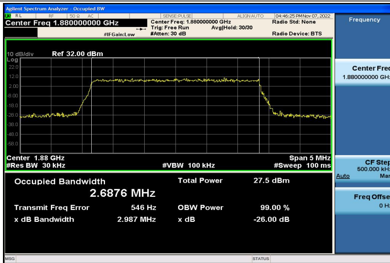
Band2-3MHz-QPSK-18900-15RB#0-2.6876
