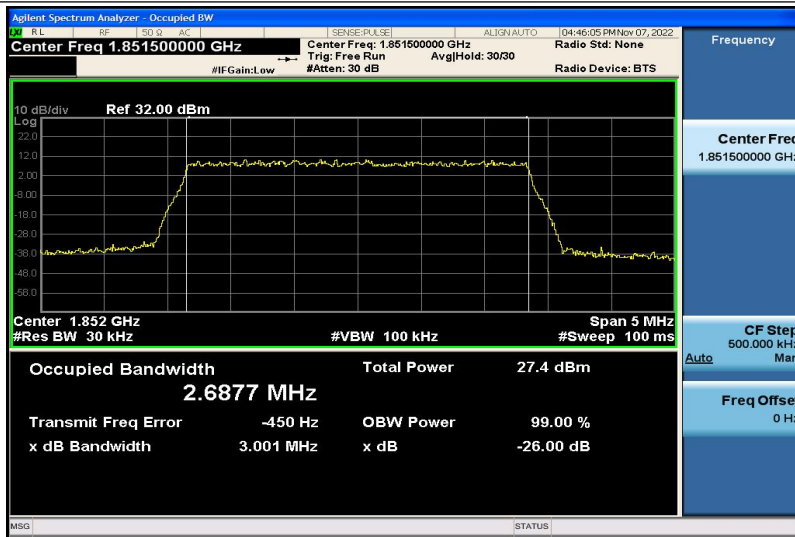
Band2-3MHz-QPSK-18615-15RB#0-2.6877
