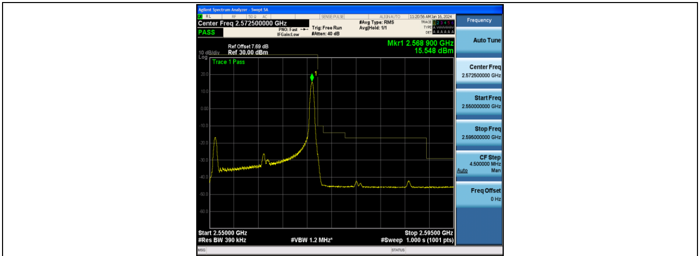
Band7_20MHz_QPSK_21350_1RB#99
