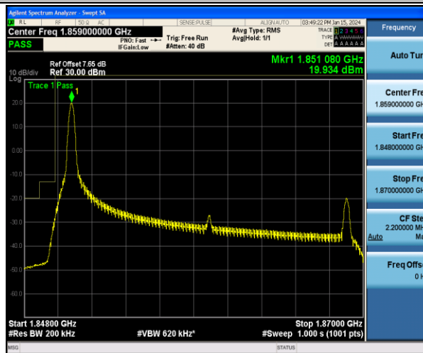
Band2_20MHz_QPSK_18700_1RB#0
