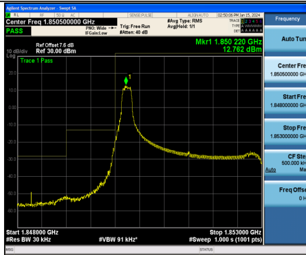
Band2_3MHz_QPSK_18615_1RB#0
