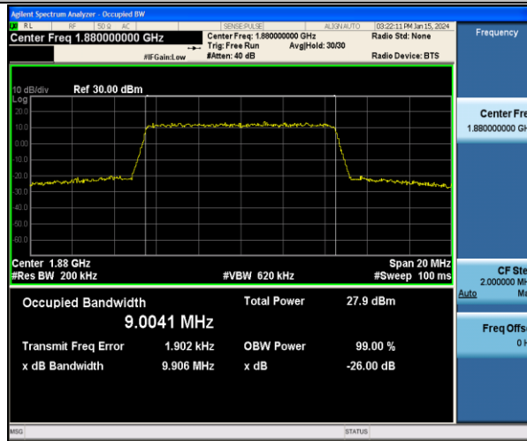
Band2-10MHz-QPSK-18900-50RB#0-PASS
