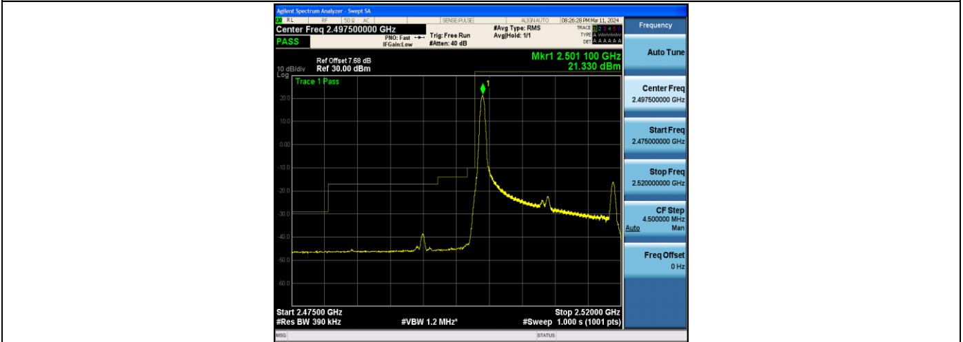
Band7_20MHz_16QAM_20850_1RB#0
