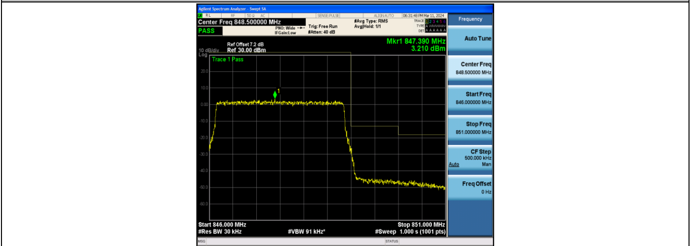
Band5_3MHz_16QAM_20635_15RB#0
