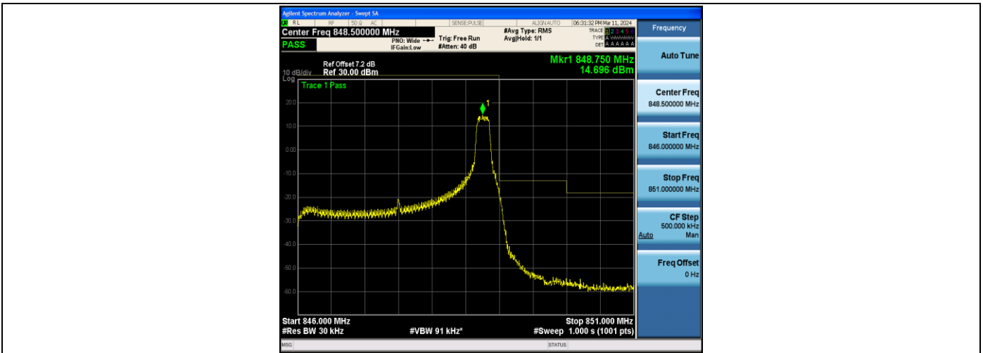
Band5_3MHz_16QAM_20635_1RB#14
