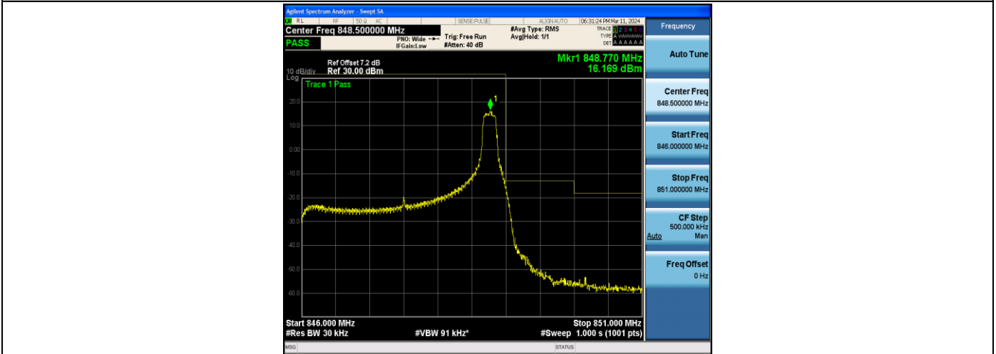
Band5_3MHz_QPSK_20635_1RB#14
