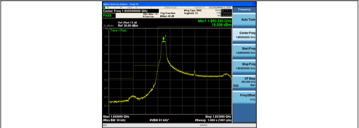
Band2_3MHz_QPSK_18615_1RB#0
