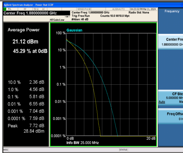
Band2-20MHz-QPSK-18900-100RB#0-PASS
