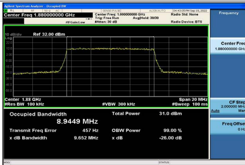
Band2-10MHz-16QAM-18900-50RB#0-8.9449
