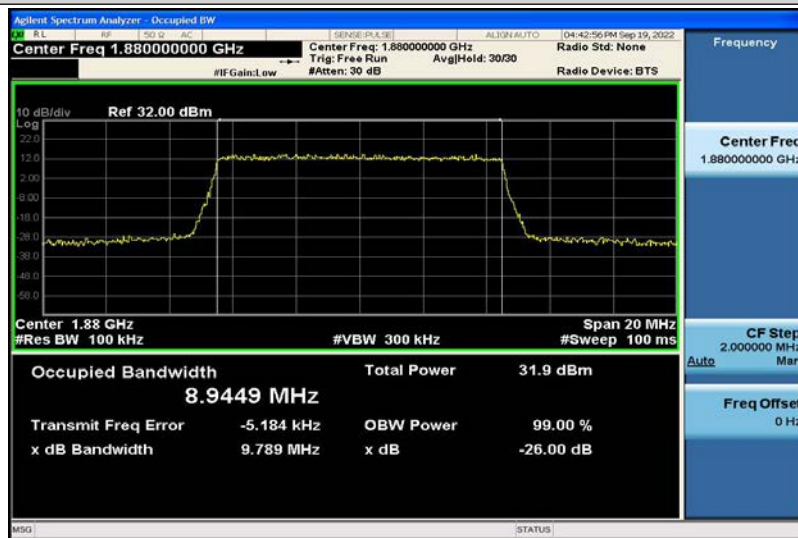
Band2-10MHz-QPSK-18900-50RB#0-8.9449
