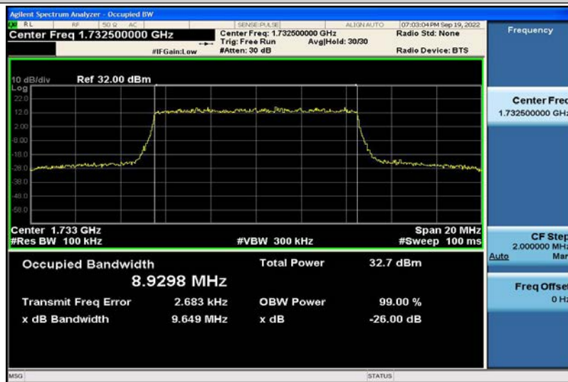
Band4-10MHz-QPSK-20175-50RB#0-8.9298
