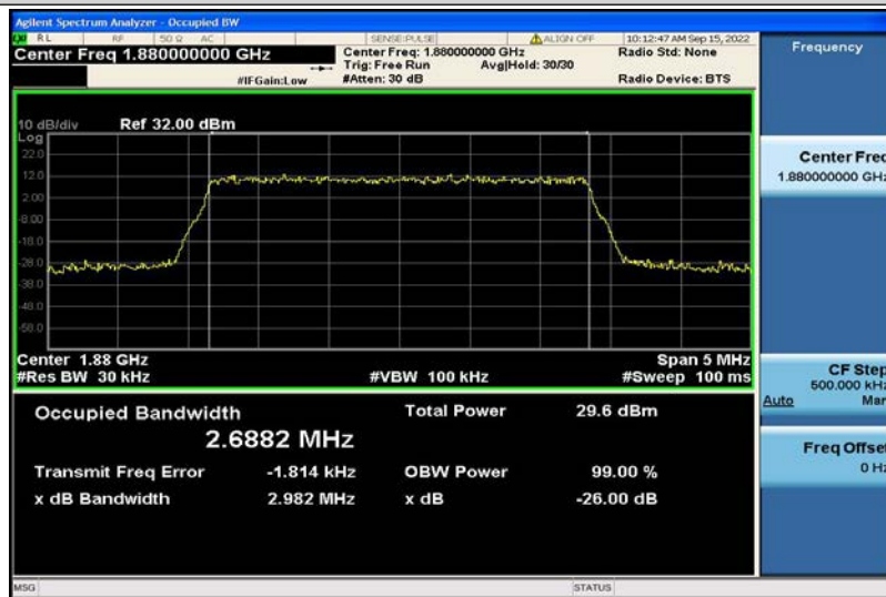
Band2-3MHz-QPSK-18900-15RB#0-2.6882
