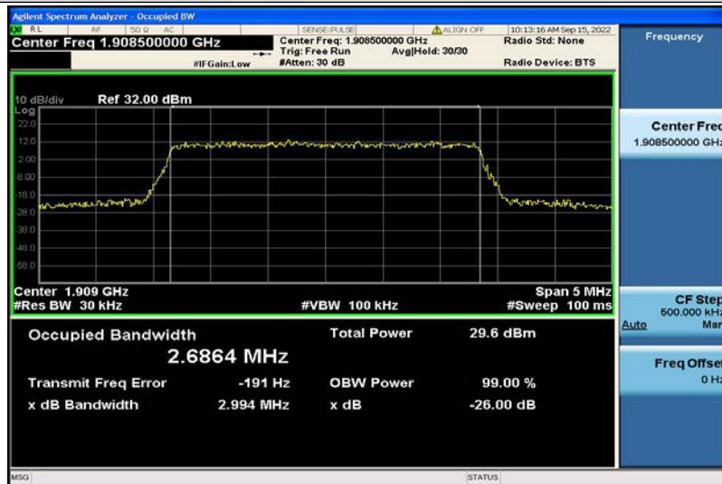
Band2-3MHz-16QAM-19185-15RB#0-2.6864
