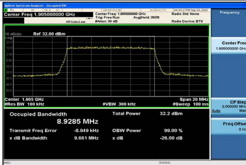
Band2-10MHz-QPSK-19150-50RB#0-8.9285
