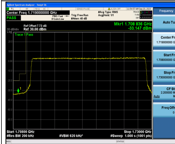
Band66_20MHz_QPSK_132072_100RB#0
