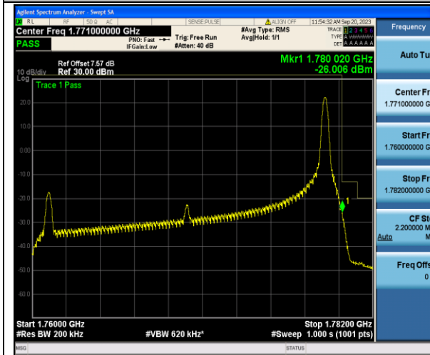
Band66_20MHz_QPSK_132572_1RB#99
