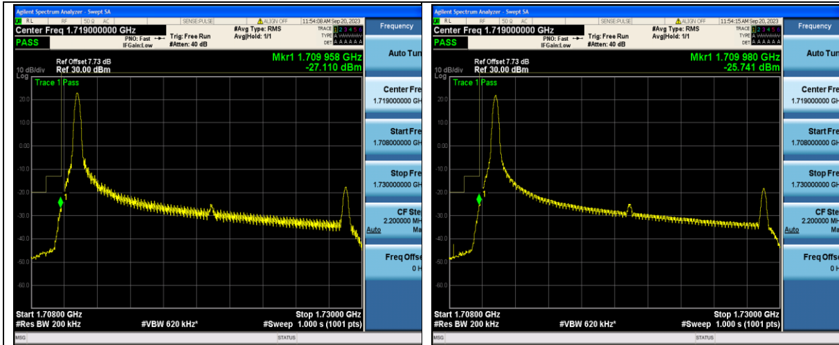
Band66_20MHz_QPSK_132072_1RB#0
