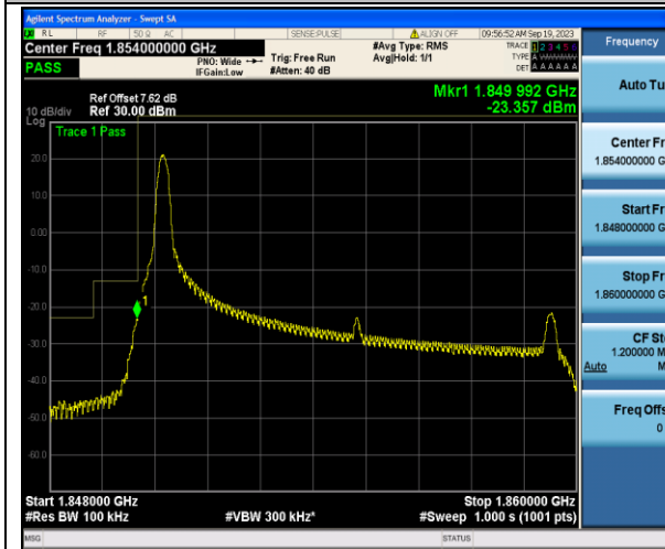
Band2_10MHz_QPSK_18650_1RB#0
