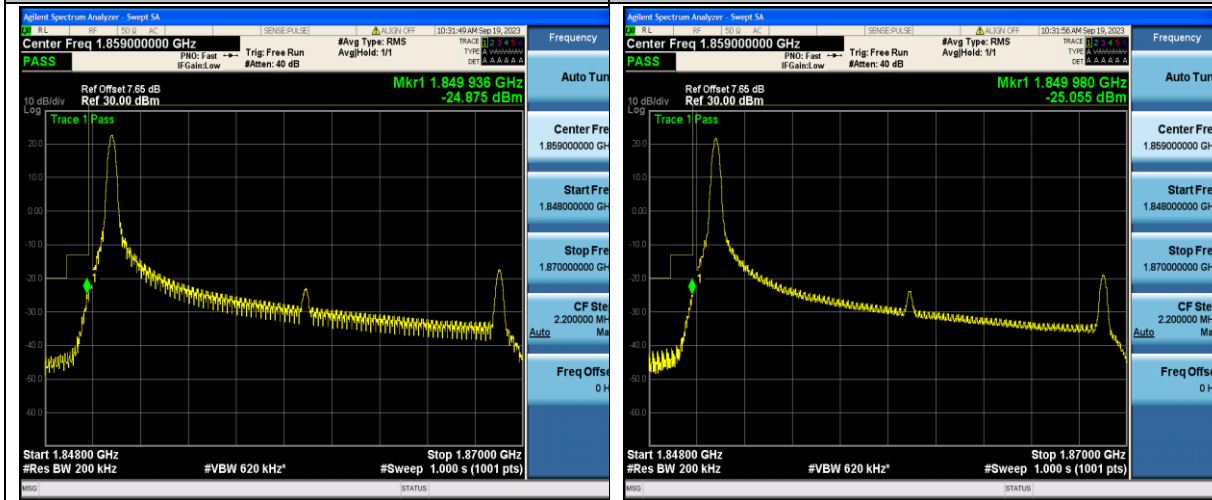
Band2_20MHz_QPSK_18700_1RB#0
