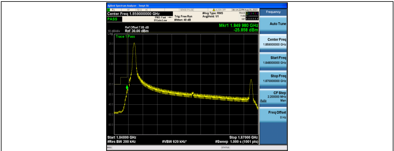
Band2_20MHz_QPSK_18700_1RB#0
