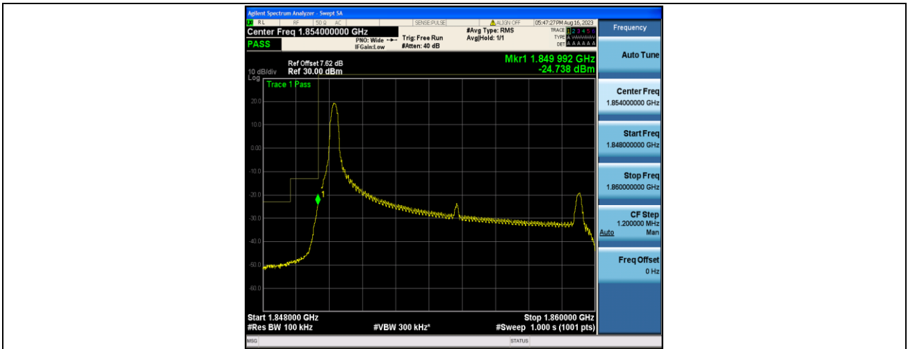
Band2_10MHz_QPSK_18650_1RB#0
