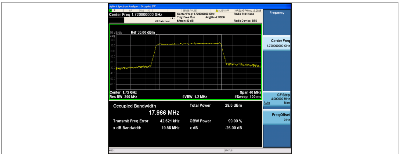
Band4-20MHz-QPSK-20050-100RB#0-PASS
