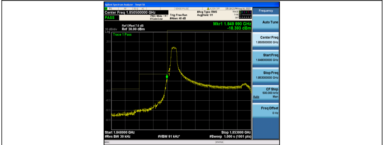
Band2_3MHz_QPSK_18615_1RB#0
