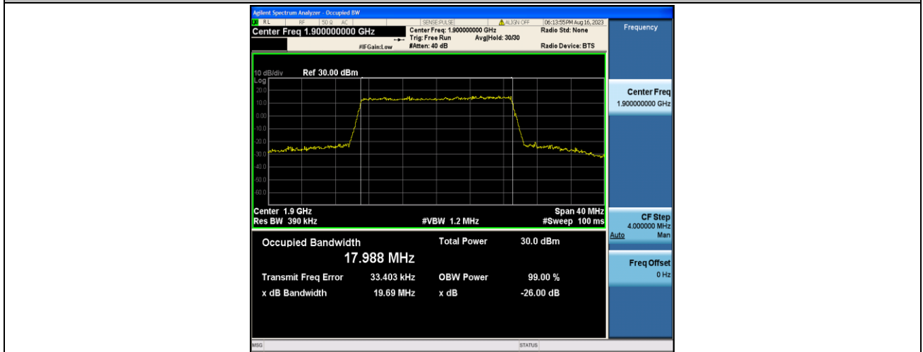
Band2-20MHz-QPSK-19100-100RB#0-PASS
