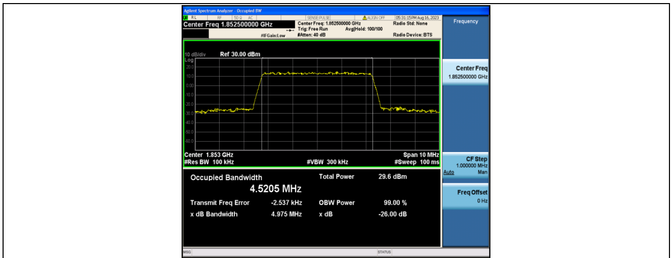
Band2-5MHz-QPSK-18625-25RB#0-PASS
