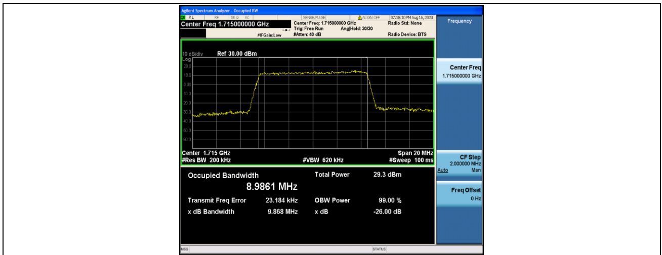
Band4-10MHz-QPSK-20000-50RB#0-PASS
