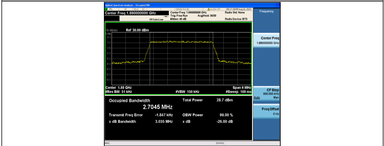
Band2-3MHz-QPSK-18900-15RB#0-PASS
