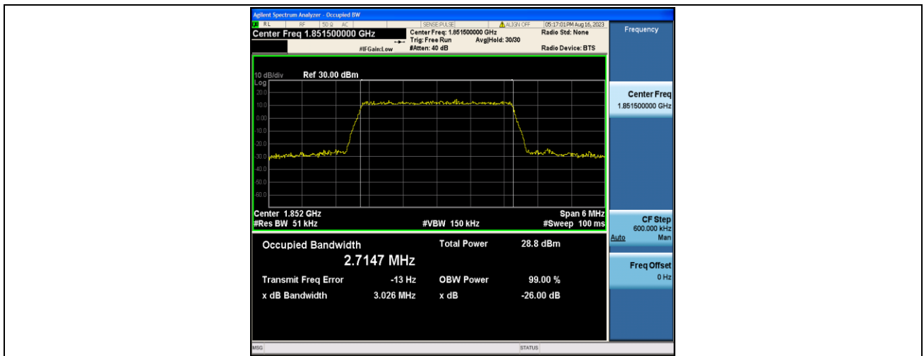
Band2-3MHz-QPSK-18615-15RB#0-PASS
