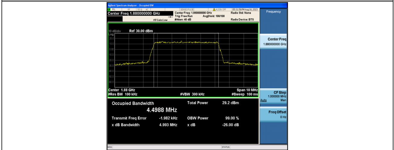
Band2-5MHz-QPSK-18900-25RB#0-PASS
