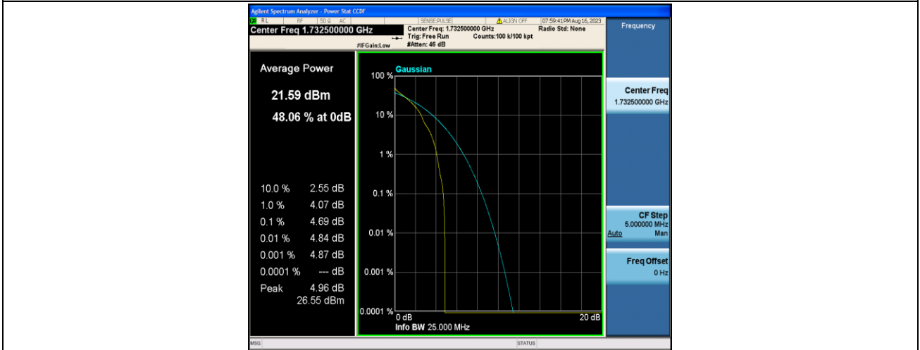
Band4-20MHz-QPSK-20175-1RB#0-PASS
