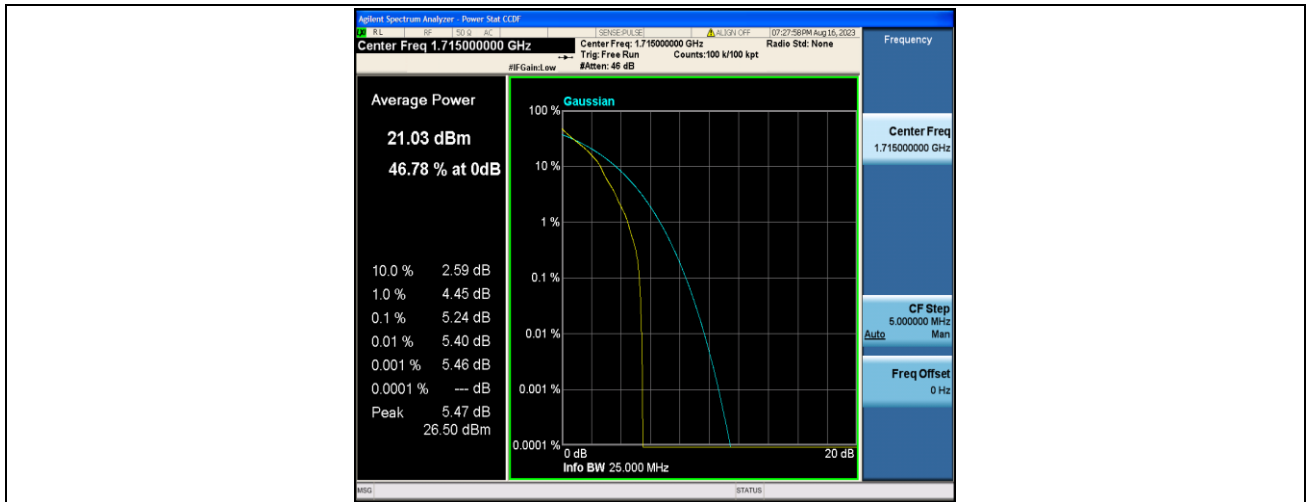
Band4-10MHz-QPSK-20000-1RB#0-PASS
