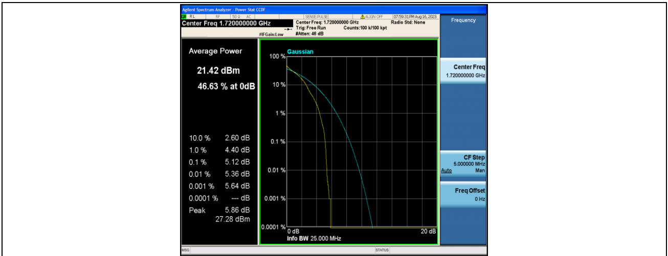
Band4-20MHz-QPSK-20050-1RB#0-PASS
