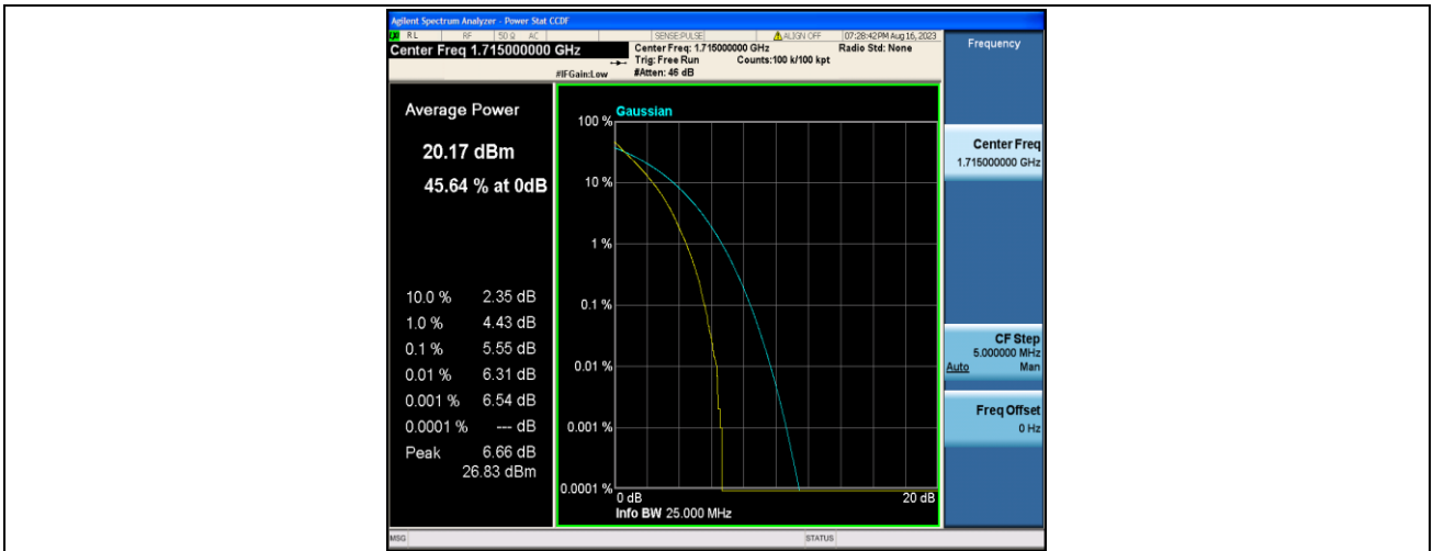
Band4-10MHz-QPSK-2000-50RB#0-PASS
