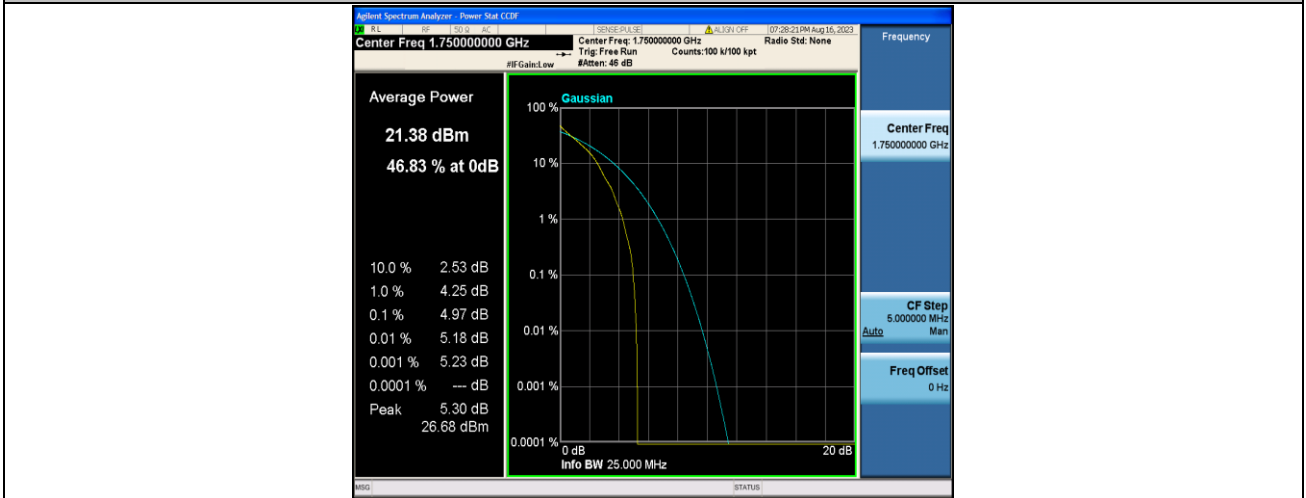
Band4-10MHz-QPSK-20350-1RB#0-PASS
