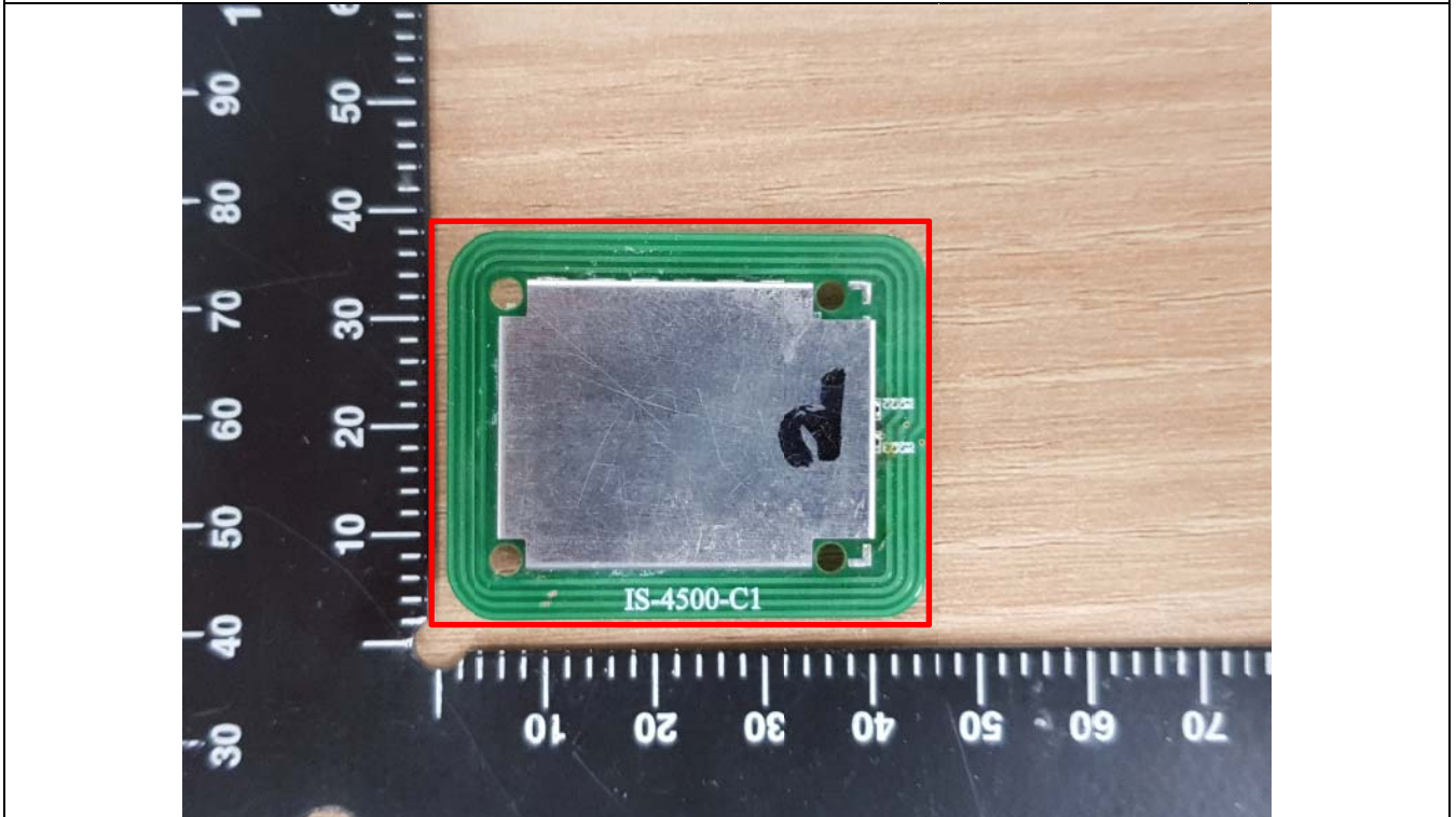
RFID Antenna
