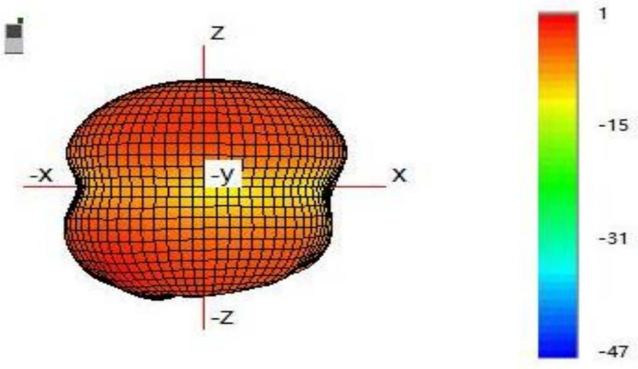
(4) 2420MHz 的 3D 方向图(单位： dBi):
