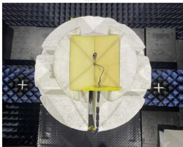
俯视图
