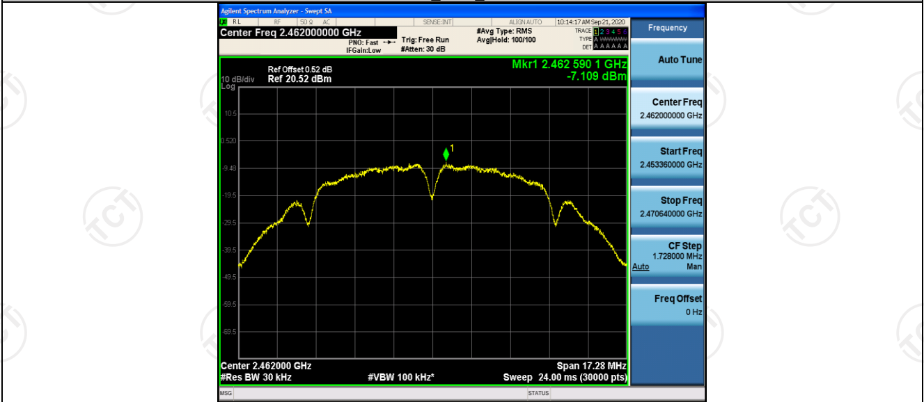
11B_Ant1_2462
