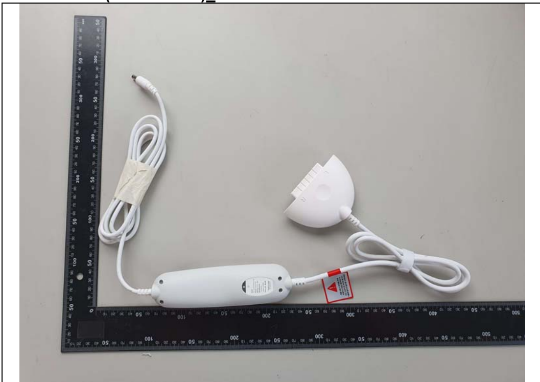
Basic Model(EME501-DP)_Rear
