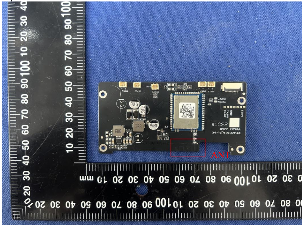
12) EUT Photo
