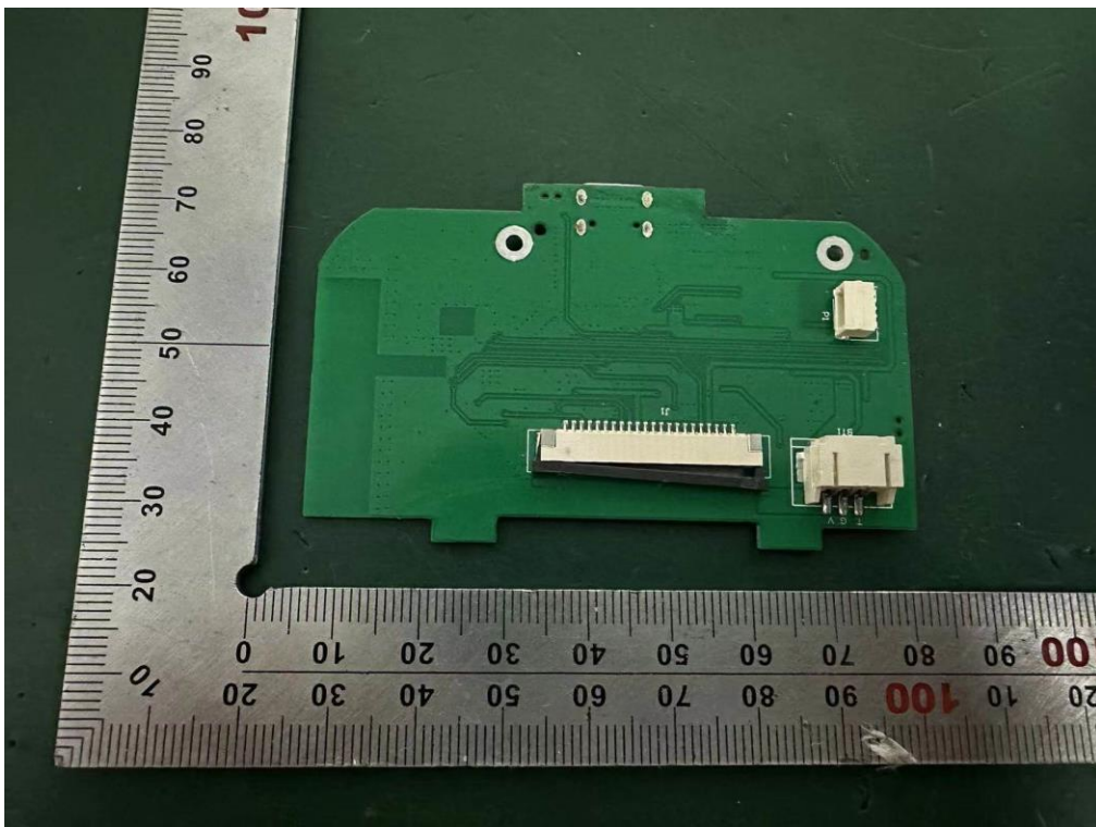
Mainboard: Q114_A 231229
