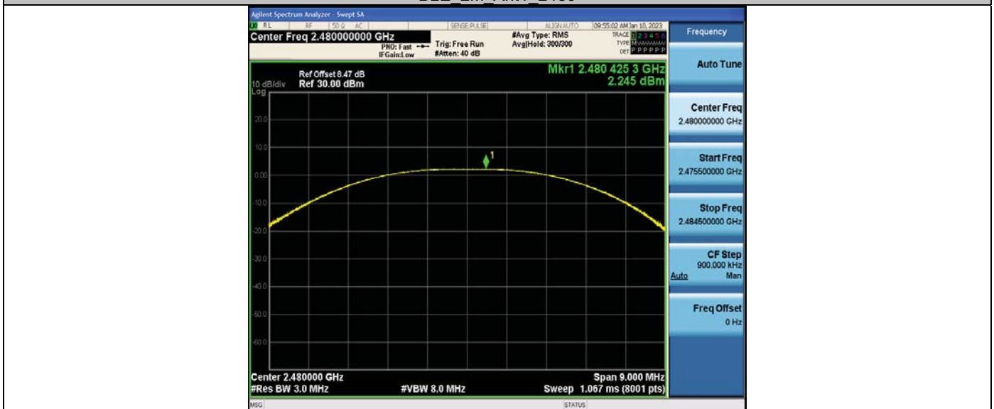
BLE 2M Ant1 2480
