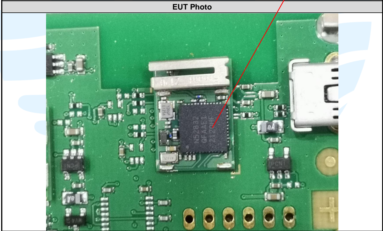
Bluetooth Module
