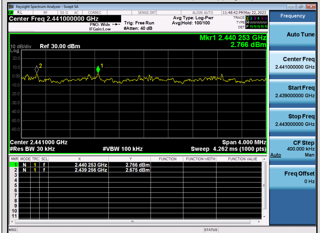
Test_Graph_BR_HOP_ANT1_NA_3Mbps_Hopping Separation
