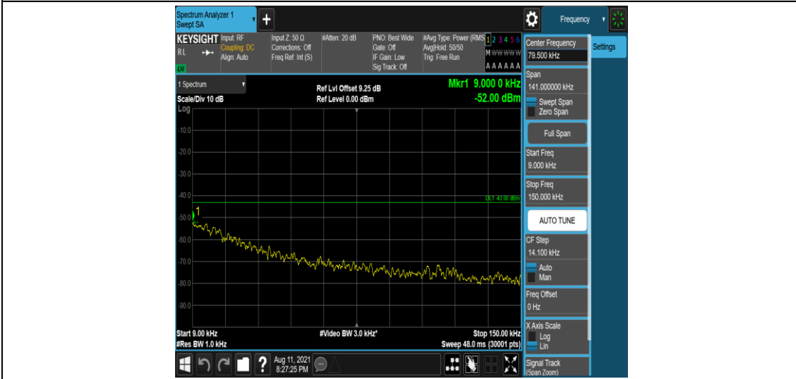
Band66-3MHz-QPSK-132322-1-0-Low-0.009-0.15--52.01-PASS
