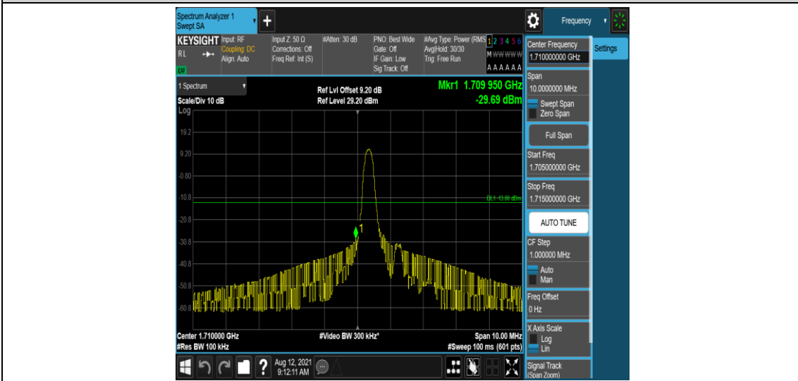
Band66-5MHz-QPSK-131997-1-0-Low--29.69-PASS
