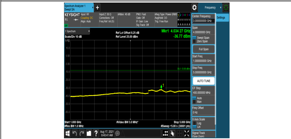
Band26-10MHz-QPSK-26840-1-0-Low-1000-5000--36.77-PASS
