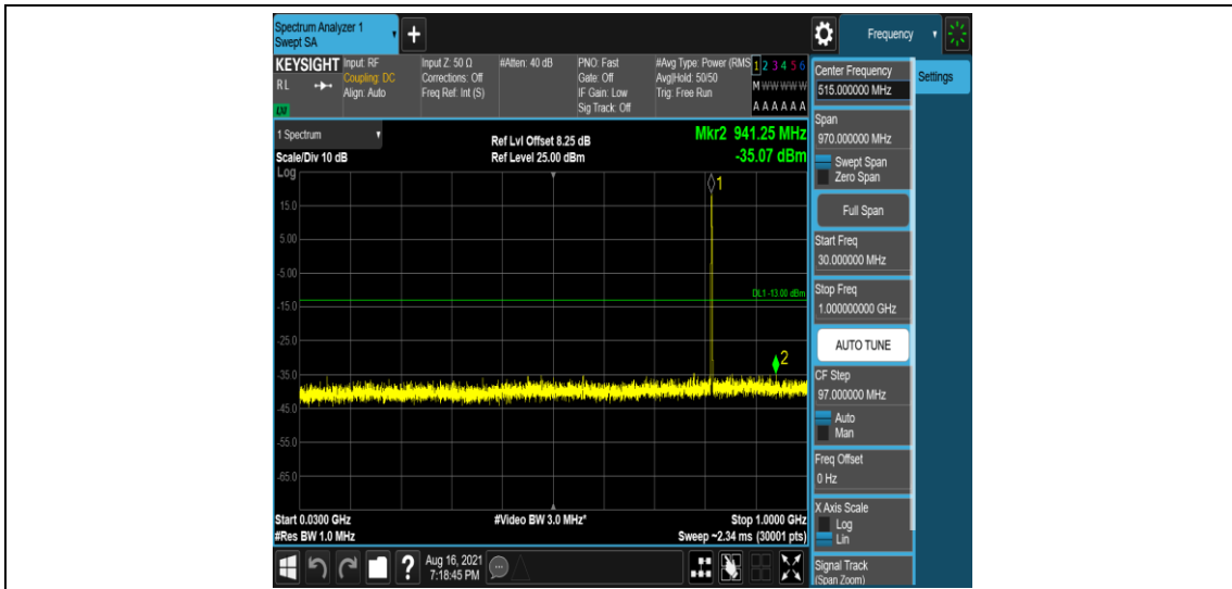
Band26-3MHz-QPSK-26740-1-0-Low-30-1000--35.07-PASS
