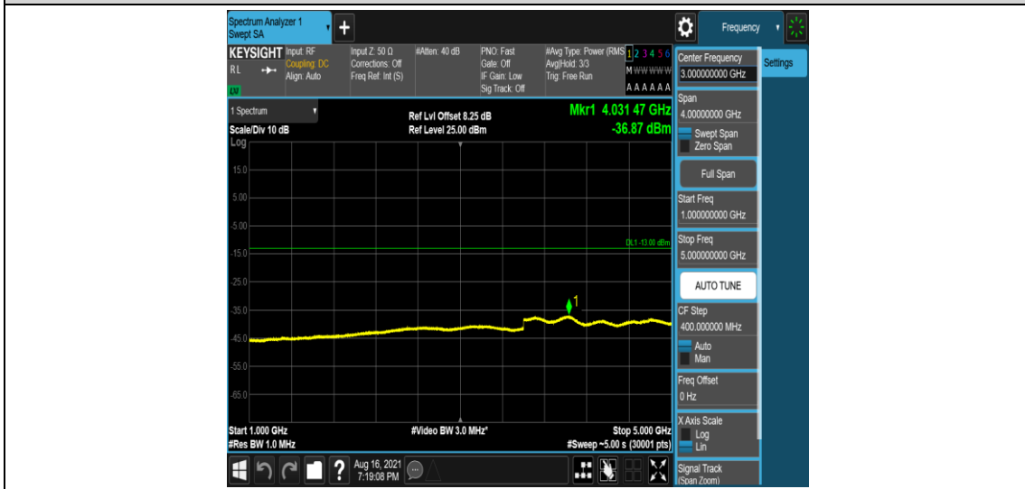
Band26-3MHz-QPSK-26740-1-0-Low-1000-5000--36.87-PASS
