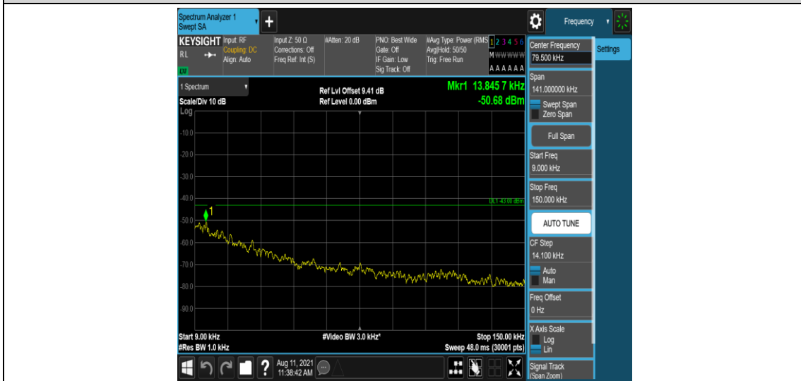
Band25-20MHz-QPSK-26365-1-0-Low-0.009-0.15--50.68-PASS
