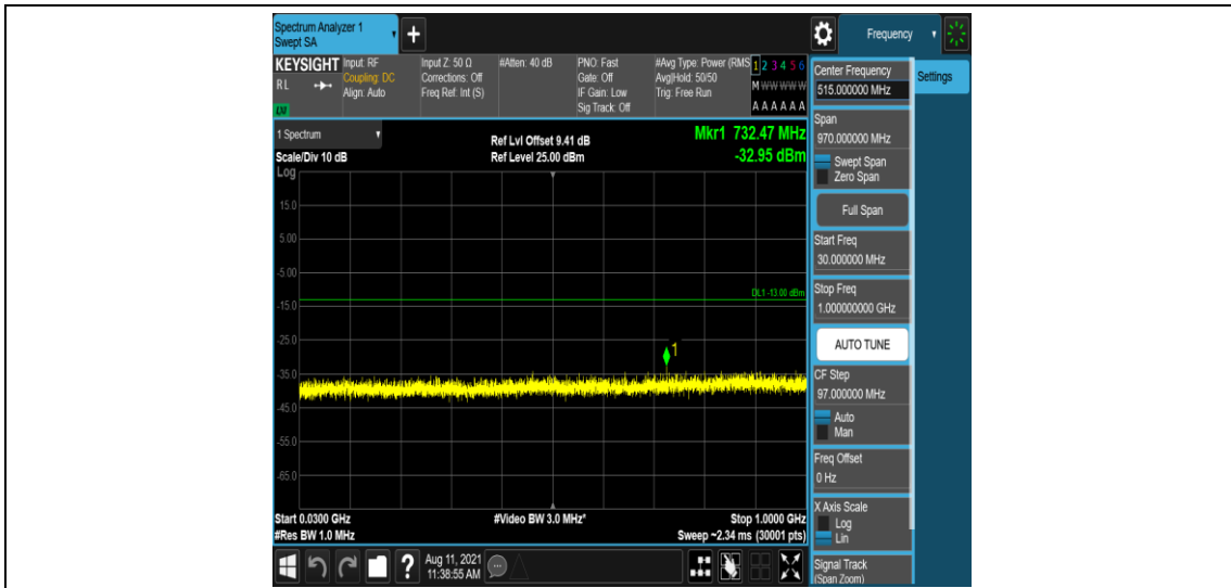
Band25-20MHz-QPSK-26365-1-0-Low-30-1000--32.95-PASS
