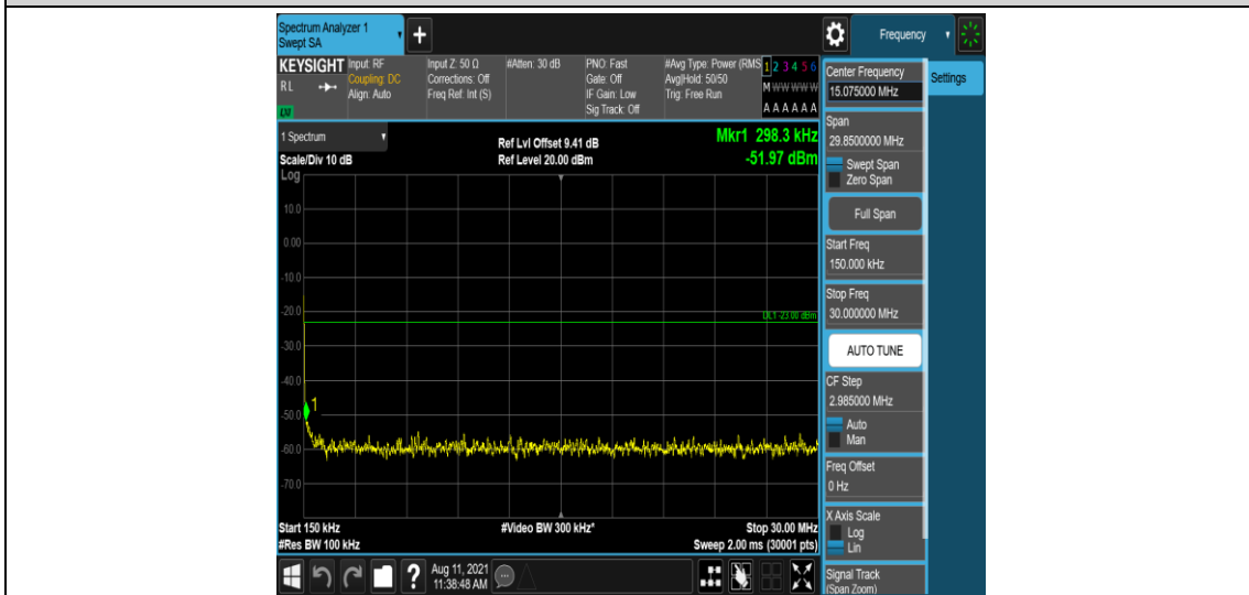
Band25-20MHz-QPSK-26365-1-0-Low-0.15-30--51.97-PASS
