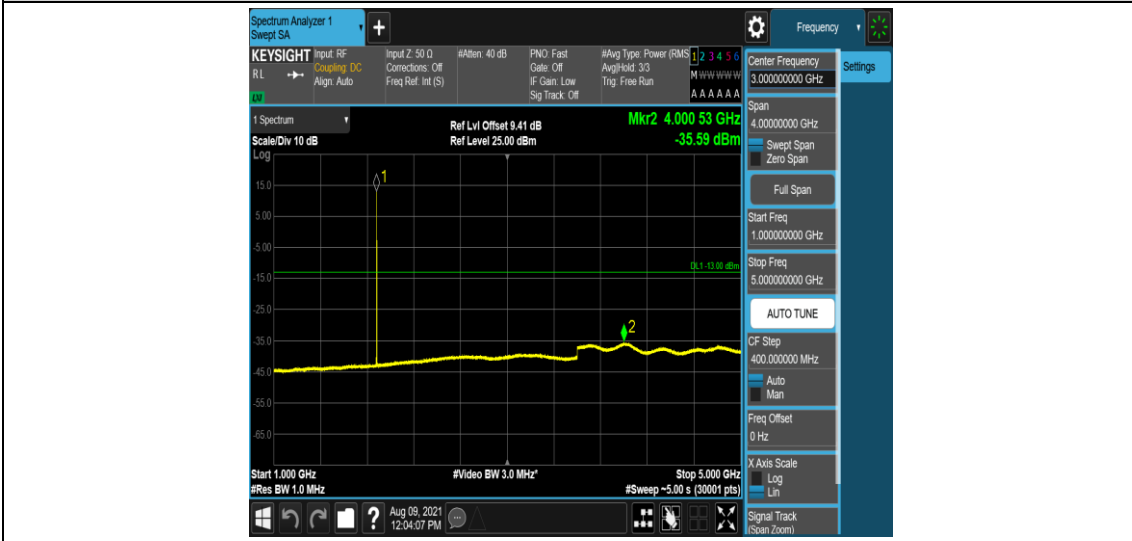
Band25-5MHz-QPSK-26365-1-0-Low-1000-5000--35.59-PASS
