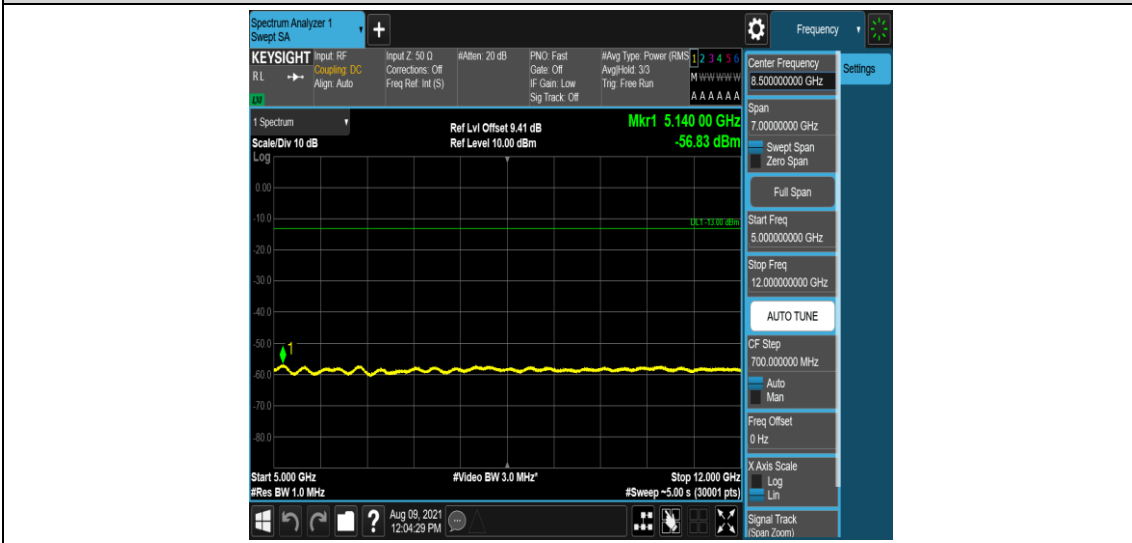
Band25-5MHz-QPSK-26365-1-0-Low-5000-12000--56.83-PASS
