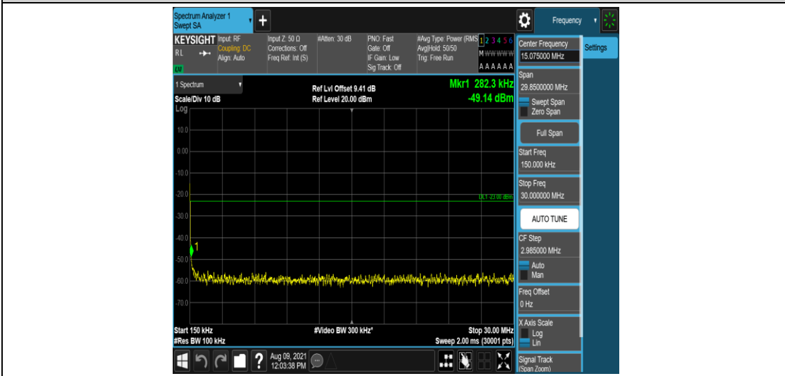
Band25-5MHz-QPSK-26365-1-0-Low-0.15-30--49.14-PASS
