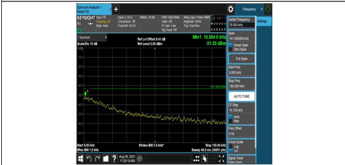
Band25-3MHz-QPSK-26365-1-0-Low-0.009-0.15--51.55-PASS
