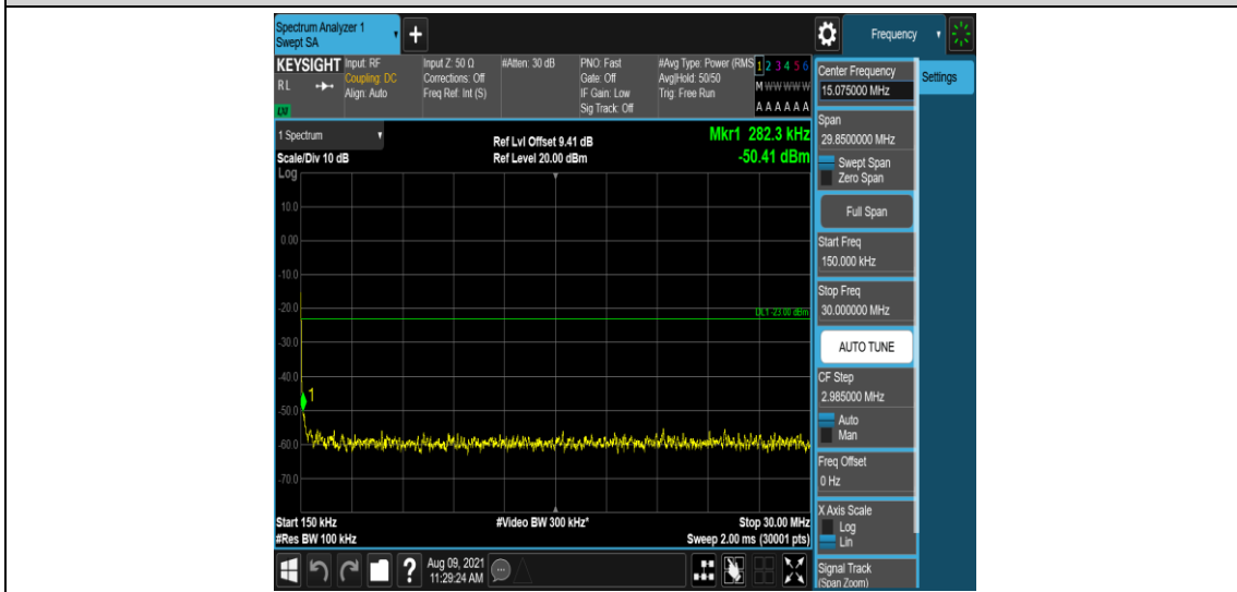
Band25-3MHz-QPSK-26365-1-0-Low-0.15-30--50.41-PASS
