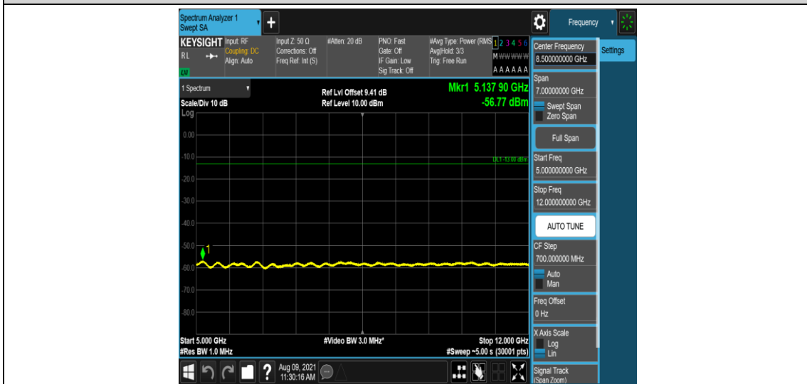
Band25-3MHz-QPSK-26365-1-0-Low-5000-12000--56.77-PASS
