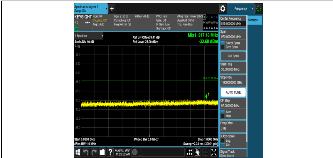
Band25-3MHz-QPSK-26365-1-0-Low-30-1000--33.68-PASS
