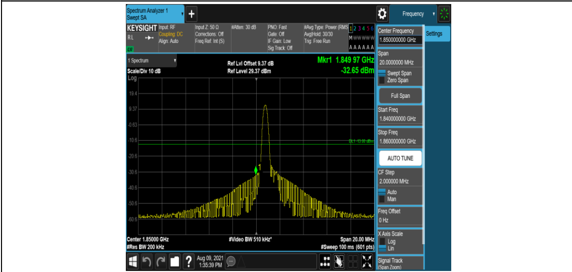
Band25-10MHz-QPSK-26090-1-0-Low--32.65-PASS
