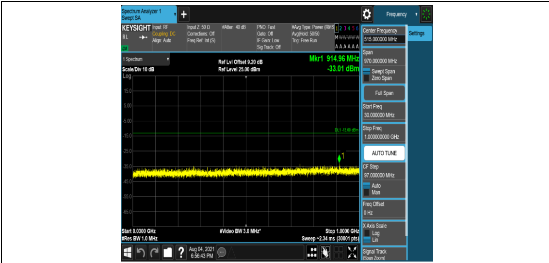
Band4-5MHz-QPSK-20175-1-0-Low-30-1000--33.01-PASS
