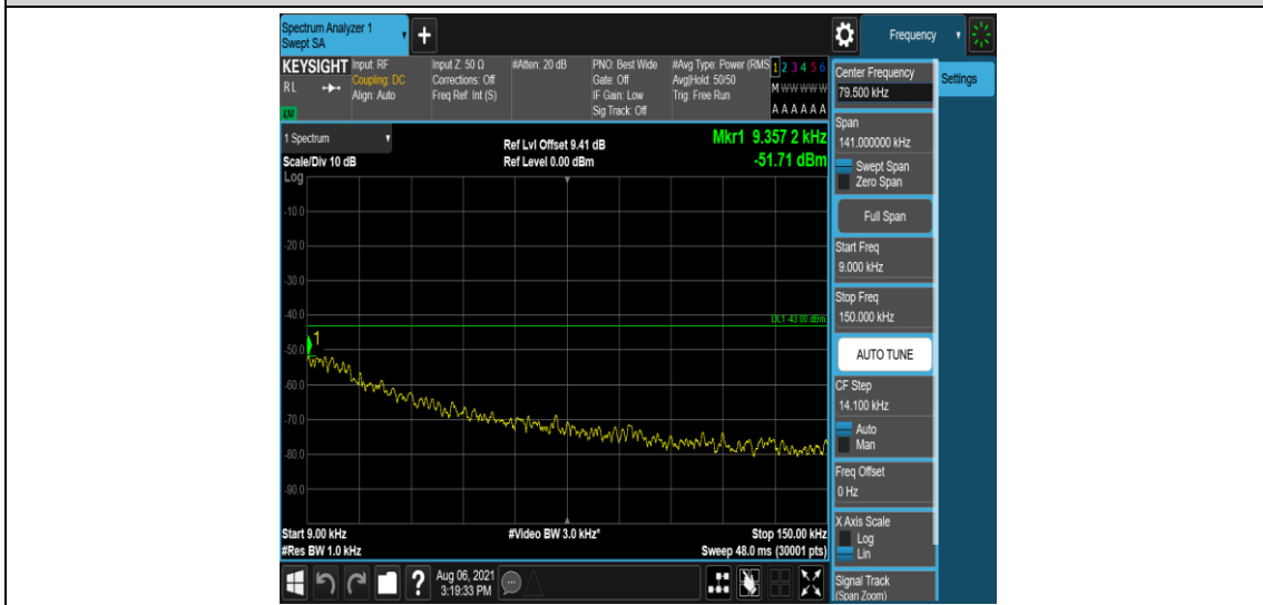
Band2-5MHz-QPSK-18900-1-0-Low-0.009-0.15--51.71-PASS
