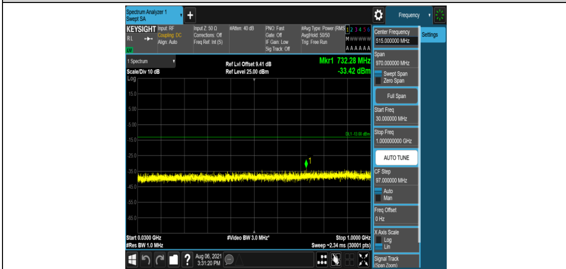
Band2-3MHz-QPSK-18900-1-0-Low-30-1000--33.42-PASS
