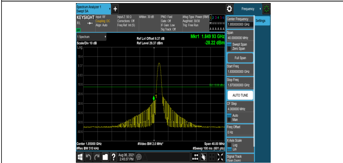
Band2-20MHz-QPSK-18700-1-0-Low--28.22-PASS
