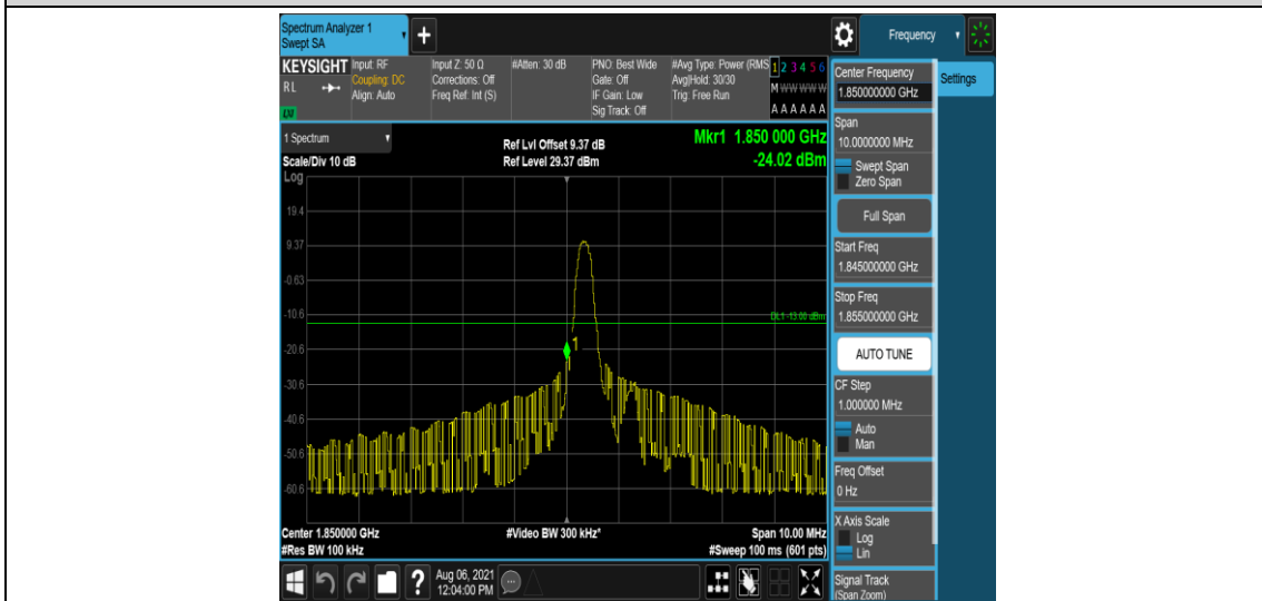
Band2-5MHz-QPSK-18625-1-0-Low--24.02-PASS
