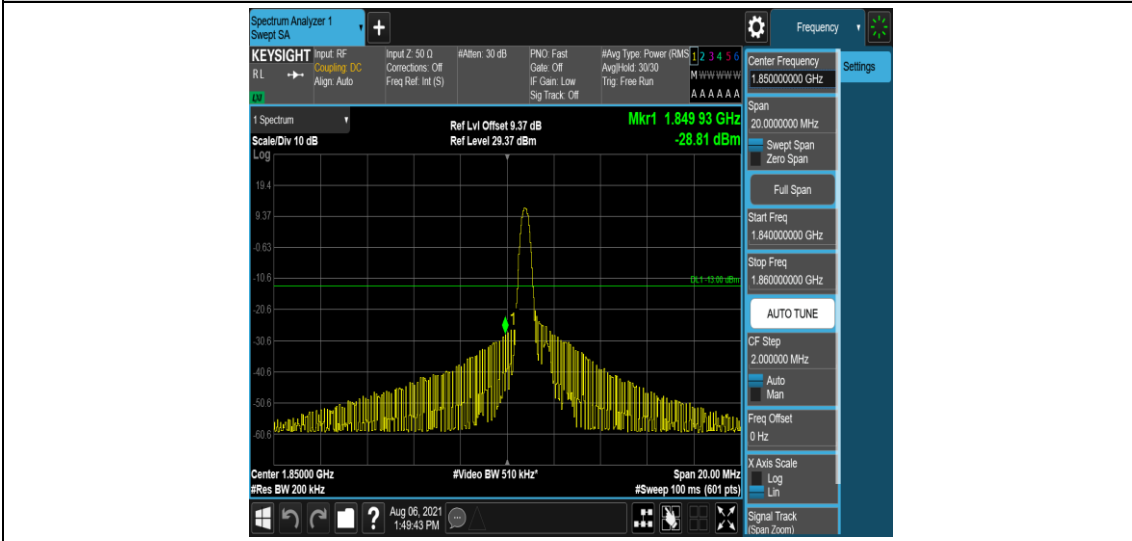
Band2-10MHz-QPSK-18650-1-0-Low--28.81-PASS
