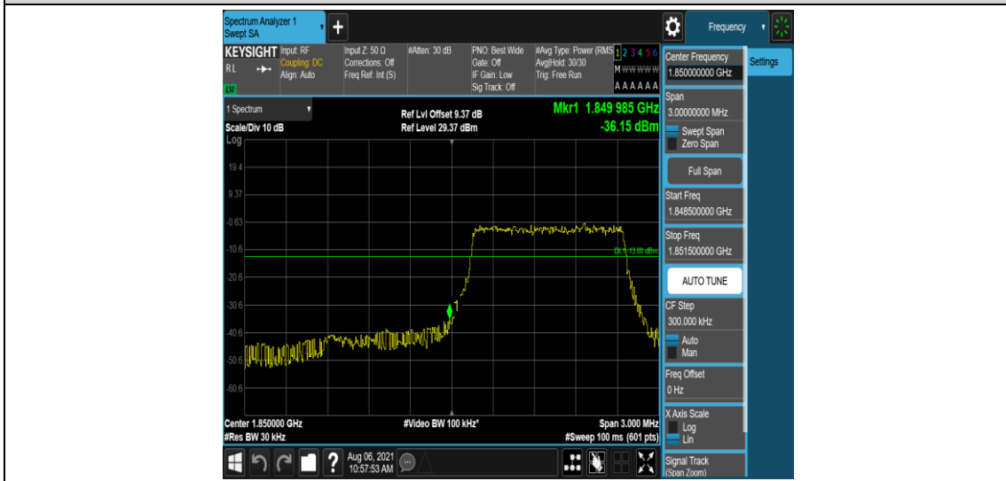
Band2-1.4MHz-QPSK-18607-1-0-Low--29.31-PASS
