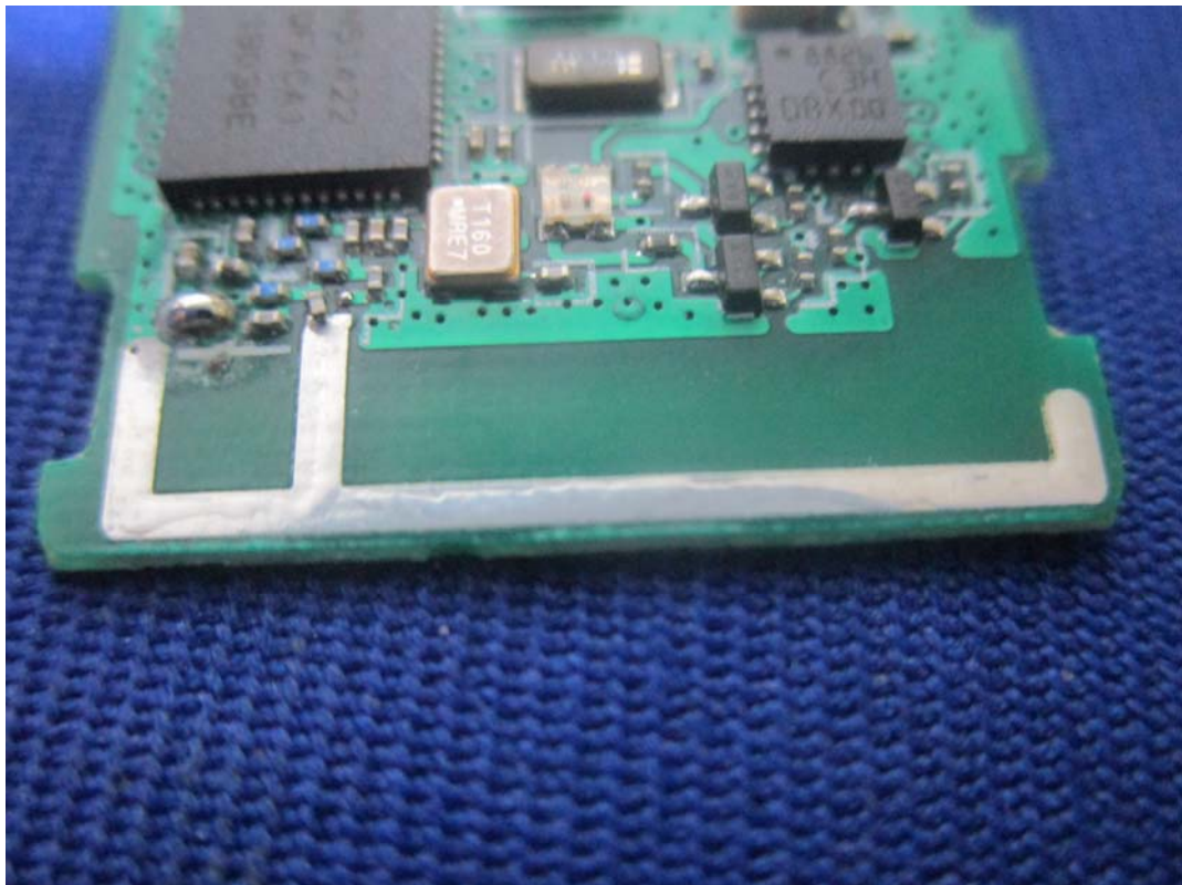
RF ANT
