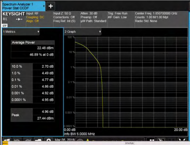
5MHz / 16QAM
