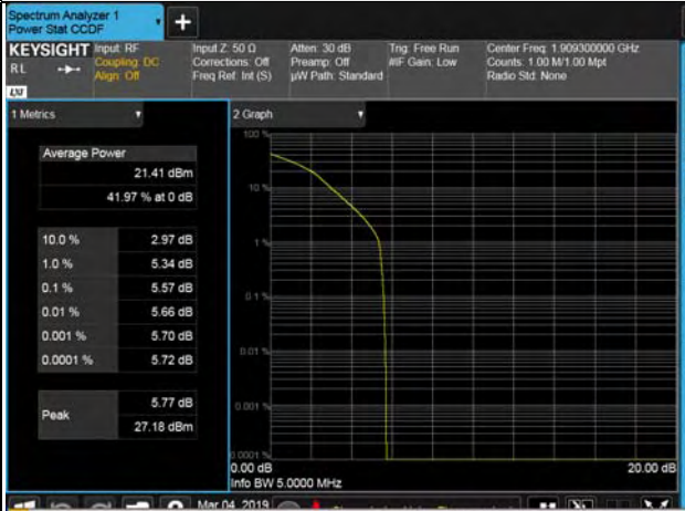
5MHz / 16QAM
