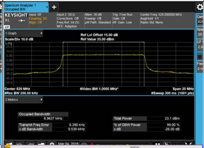
10MHz / QPSK
