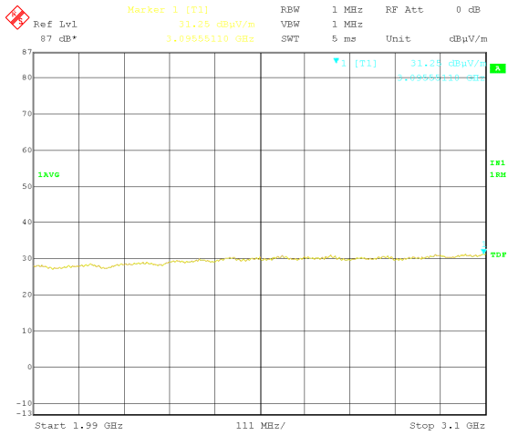
Horizontal(1 990-3 100 MHz)
