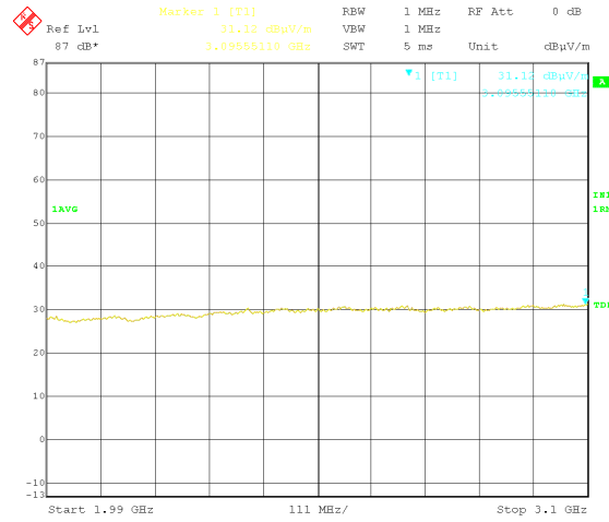
Vertical(1 990-3 100 MHz)
