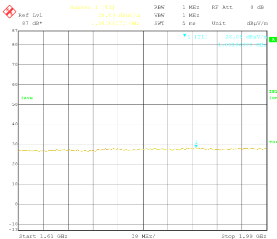
Horizontal(1 610-1 990 MHz)
