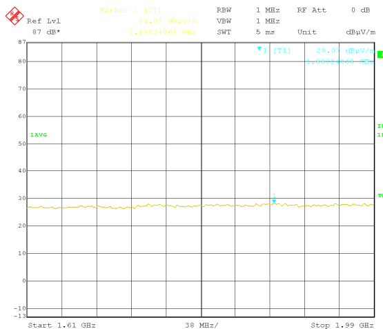
Vertical(1 610-1 990 MHz)
