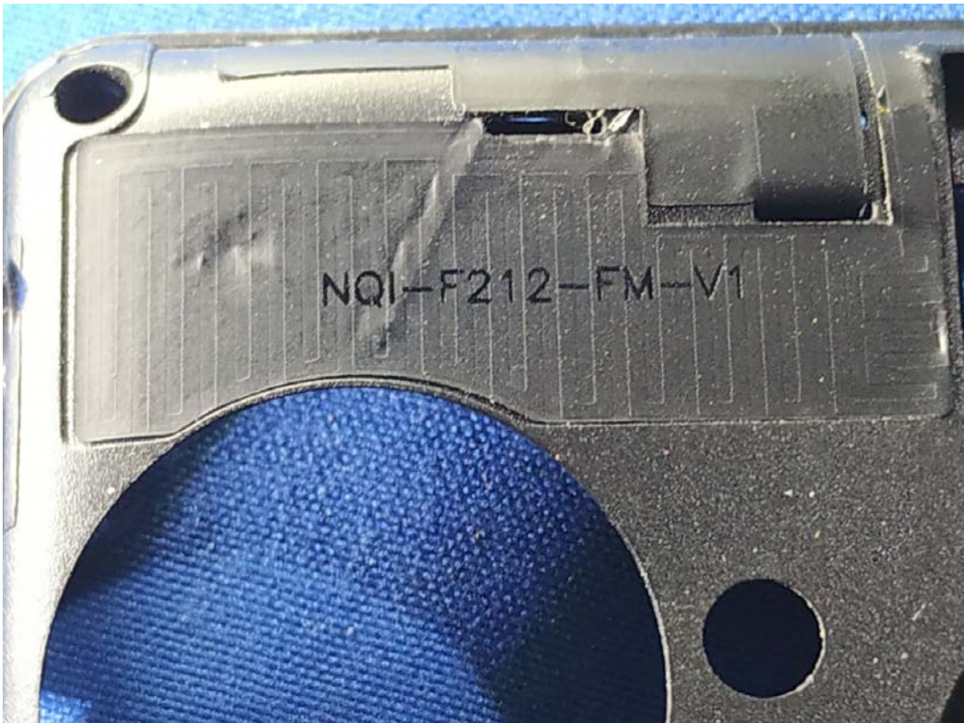
FM ANT
