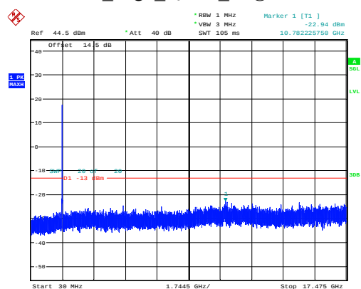
15MHz High QPSK 75@0 -22.94dBm
