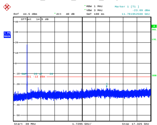
15MHz Middle QPSK 75@0 -23.09dBm
