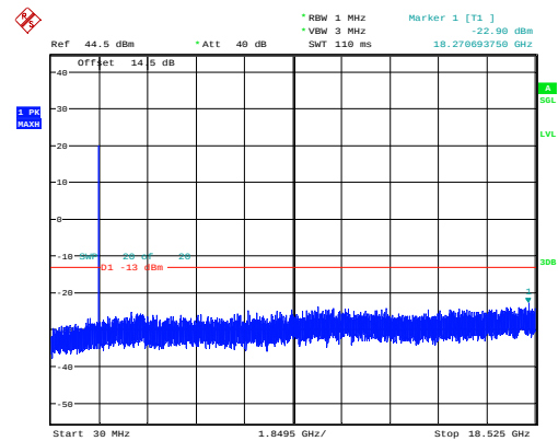
5MHz_Low_QPSK_25@0 -22.90dBm
