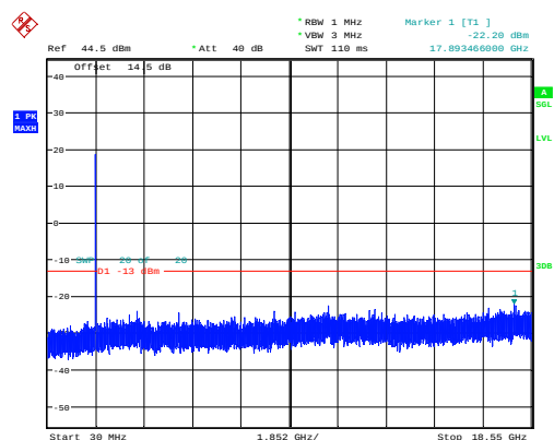
10MHz_Low_QPSK_50@0 -22.20dBm
