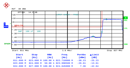
3MHz_Low_16QAM_15@0
