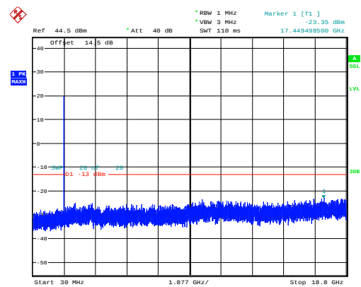
5MHz_Middle_QPSK_25@0 -23.35dBm
