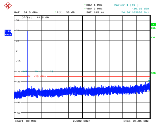
10MHz_Low_QPSK_50@0 -30.16dBm
