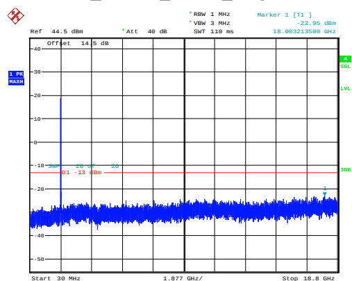
10MHz Middle QPSK 50@0 -22.95dBm
