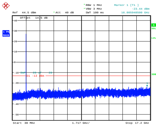
20MHz_Low_QPSK_1@0 -23.44dBm
