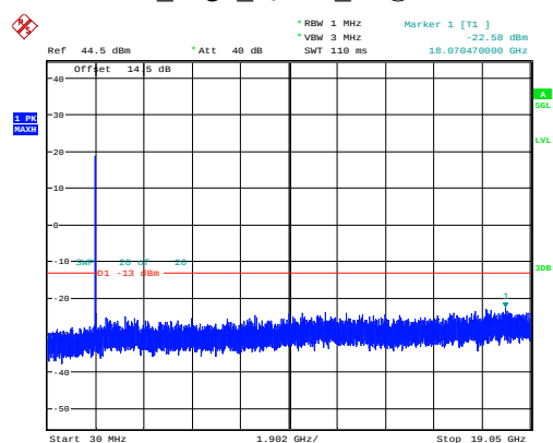
10MHz High QPSK 50@0 -22.58dBm
