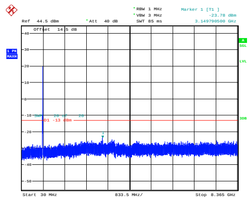
10MHz_Middle_QPSK_50@0 -23.78dBm
