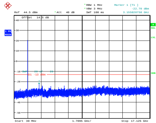
5MHz_Low_QPSK_25@0 -22.70dBm
