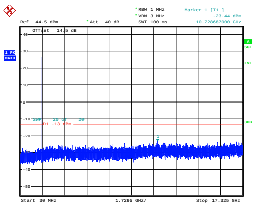
5MHz_Middle_QPSK_1@0 -23.44dBm
