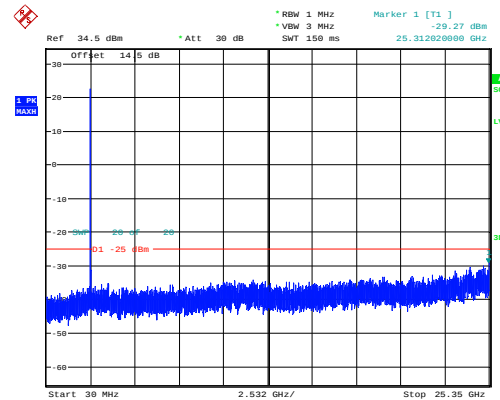
5MHz_Middle_QPSK_25@0 -29.27dBm
