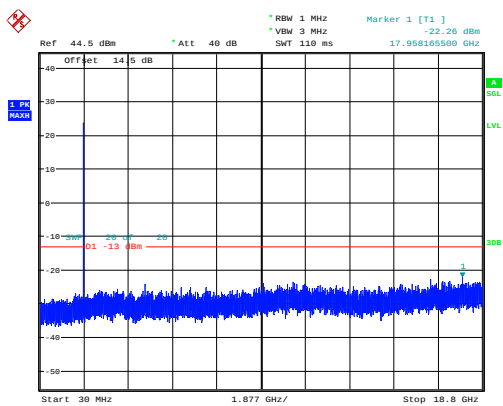
5MHz_Middle_QPSK_1@0 -22.26dBm
