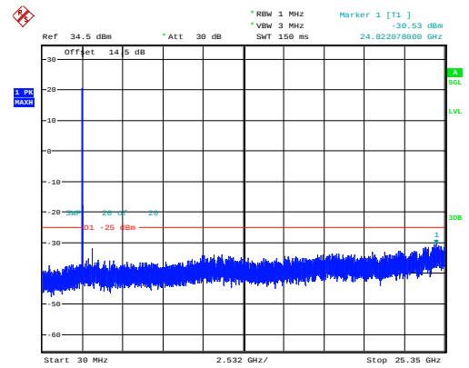
10MHz_Middle_QPSK_50@0 -30.53dBm
