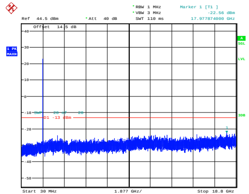
1.4MHz_Middle_QPSK_6@0 -22.56dBm
