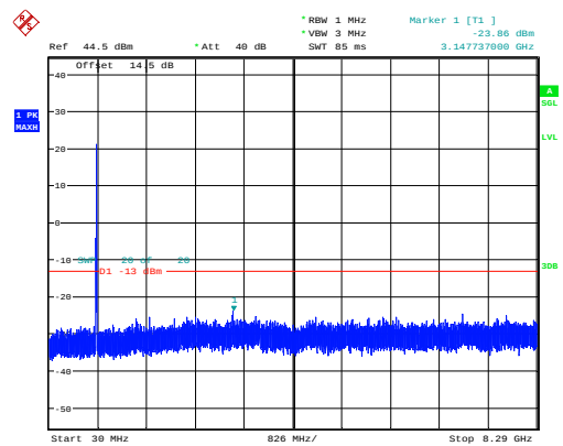
10MHz_Low_QPSK_50@0 -23.86dBm
