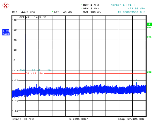
5MHz_Low_QPSK_1@0 -23.08dBm
