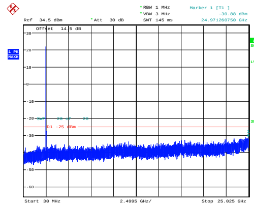
5MHz_Low_QPSK_25@0 -30.88dBm
