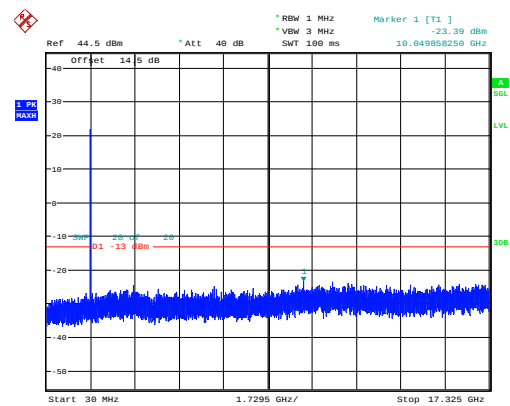
5MHz_Middle_QPSK_25@0 -23.39dBm
