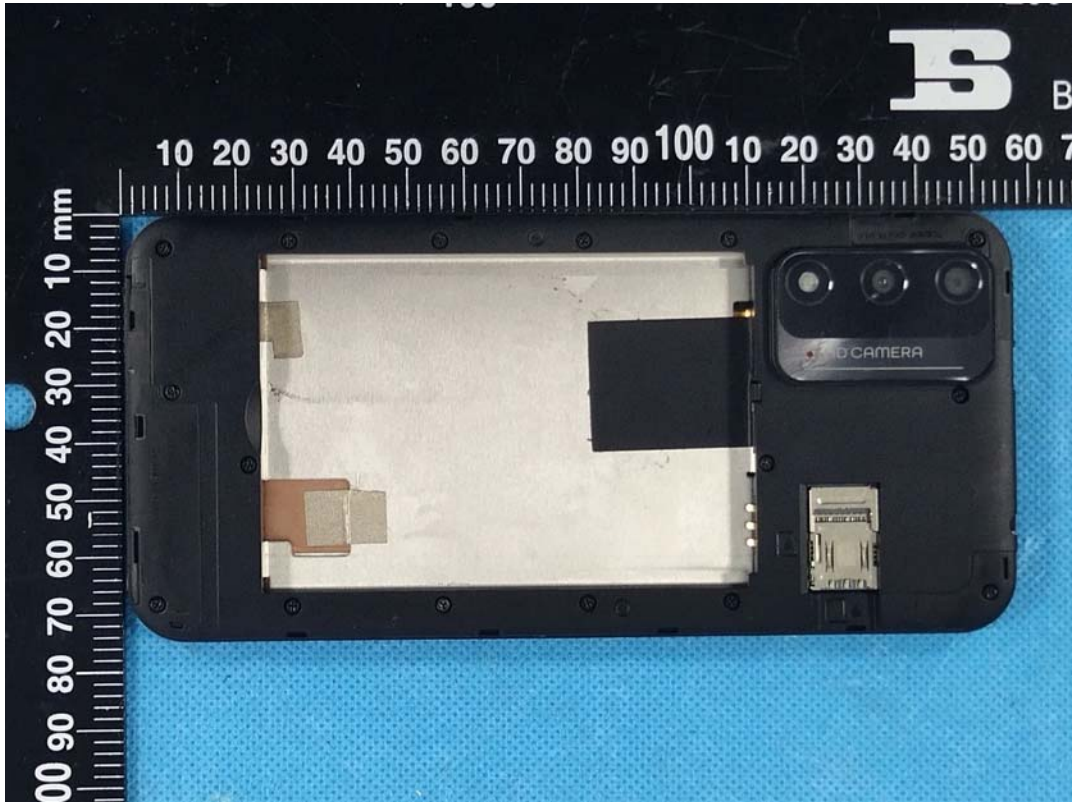
GPS/WiFi/BT Antenna
